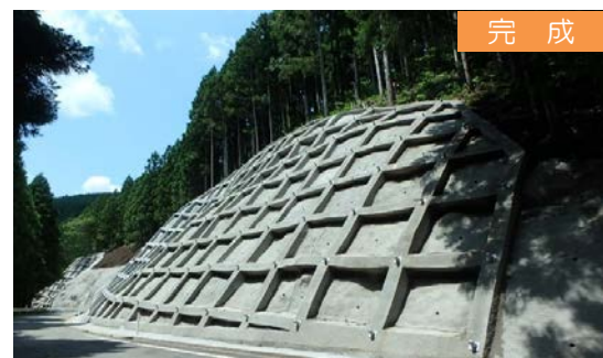
下羽沢災害防除工事（H29.9完成）
