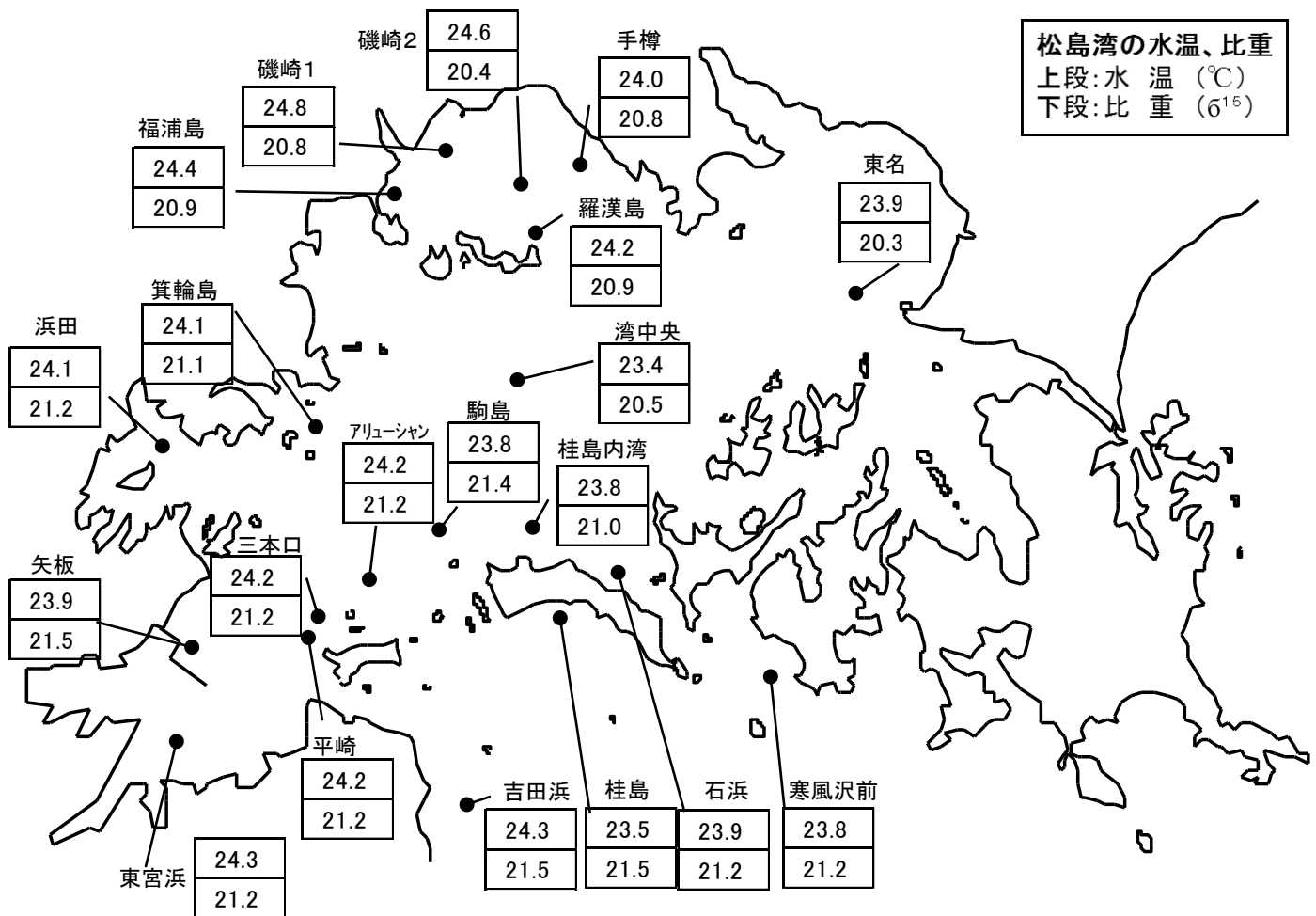
図1 松島湾の水温・比重
