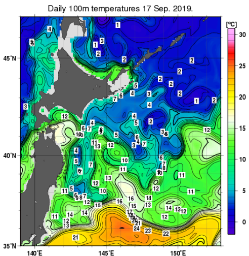
100 m深水温
