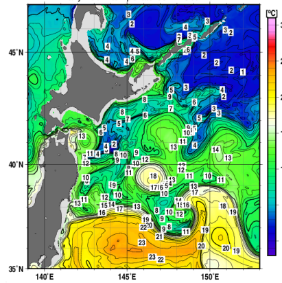
100 m深水温
