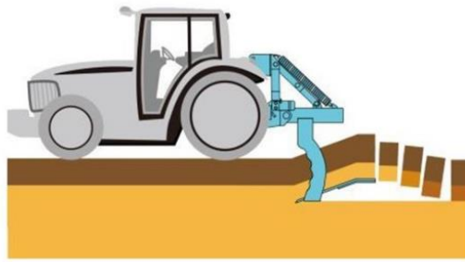
左：トラクタ走行と土塊の持上げ・破碎・落下の状況、右：破碎溝の構築方法
