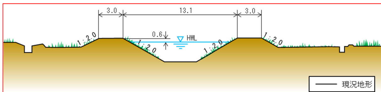
図 29 横断図(多田川合流点から 4, 200m)
