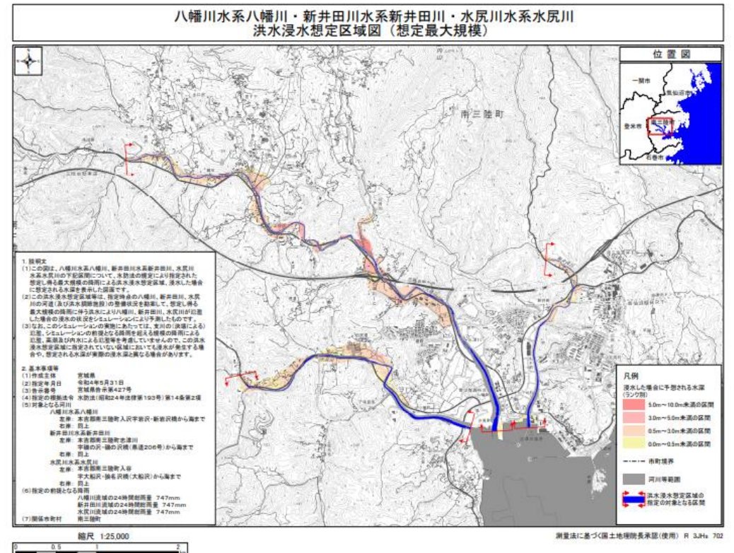
南三陸町 八幡川・新井田川・水尻川浸水想定区域図
