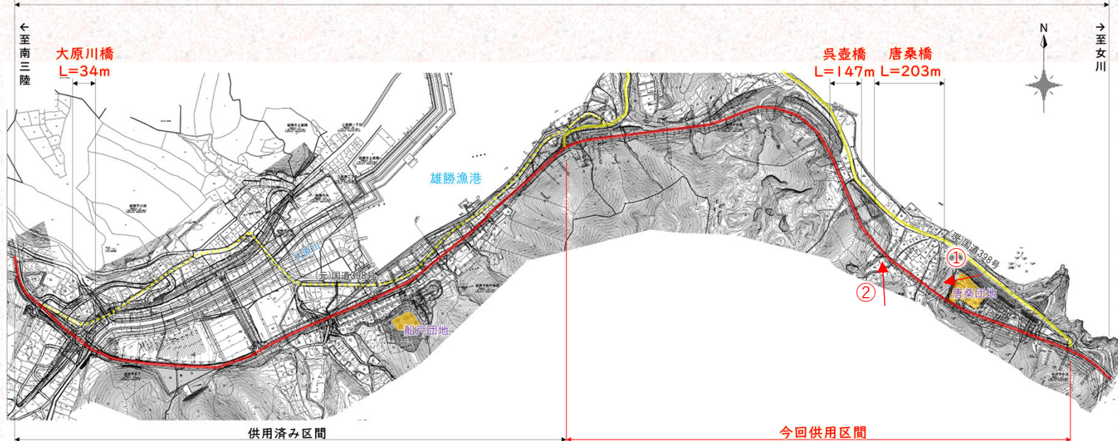
【平面図】
