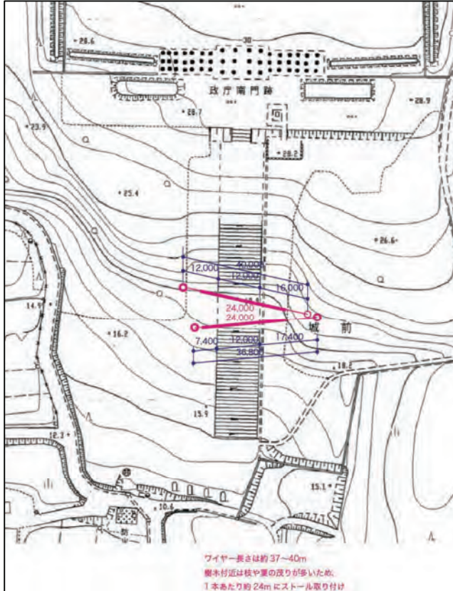
ストール用ワイヤー設置箇所 (40mワイヤー2本)
