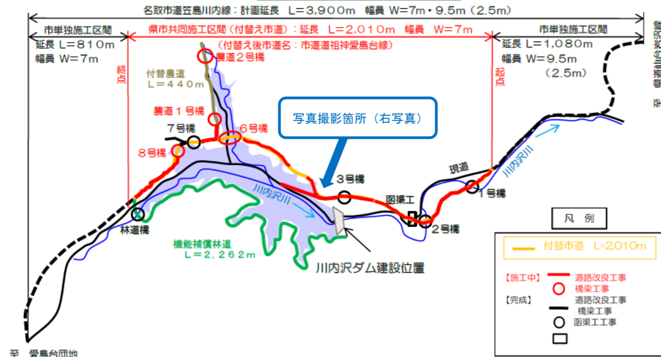
川内沢ダム建設事業全体平面図
