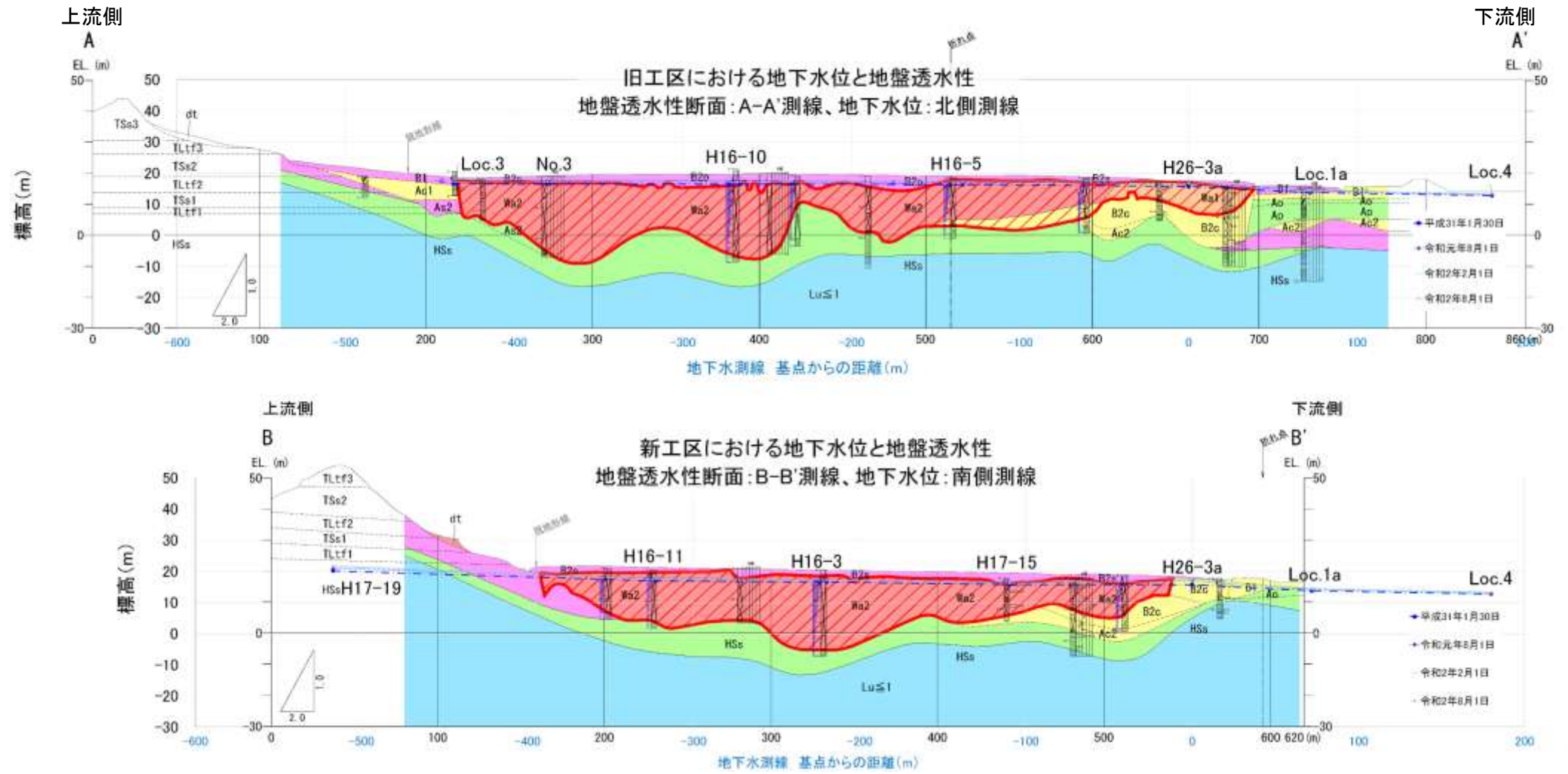
図5-13 令和2年度上半期のの上流側～下流側にかけての水位標高変化（地盤透水性断面図）
