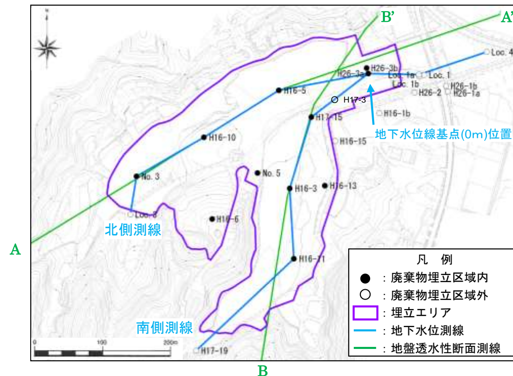
図5-14 令和2年度上半期のの上流側～下流側にかけての水位標高変化（平面図）
