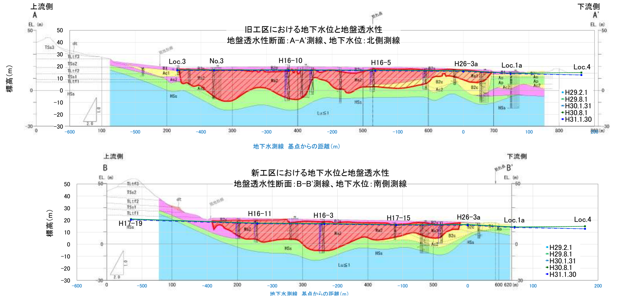
図5-13 平成30年度下期の上流側～下流側にかけての水位標高変化(地盤透水性断面図)
