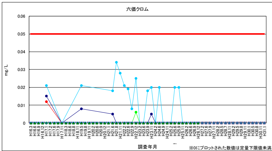
図 3-8 六価クロム（浸透水・地下水）
