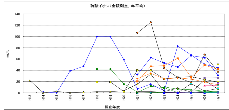
図 2-47 硫酸イオン（浸透水）
