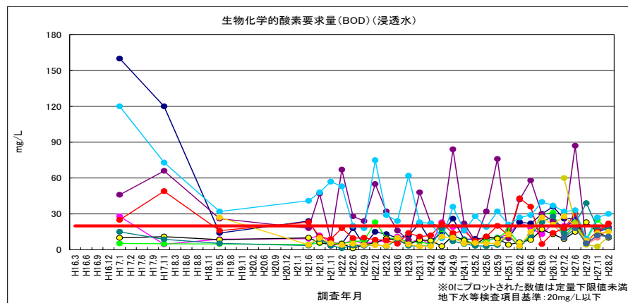
図 2-31 生物学的酸素要求量(BOD)(浸透水)
