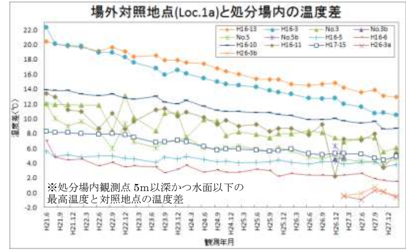
図 2-54 処分場内高温部と対照地点 (Loc.1a) との温度差の変化
