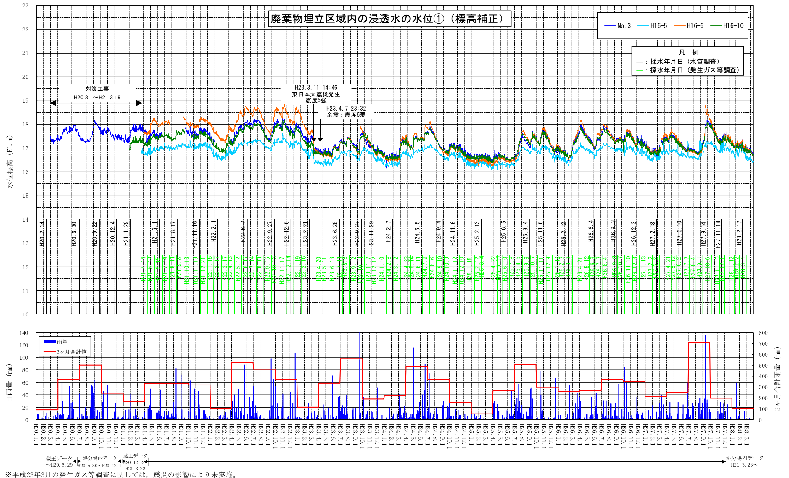
図 2-59 地下水位経時変化図（廃棄物埋立区域内の浸透水の水位①）
