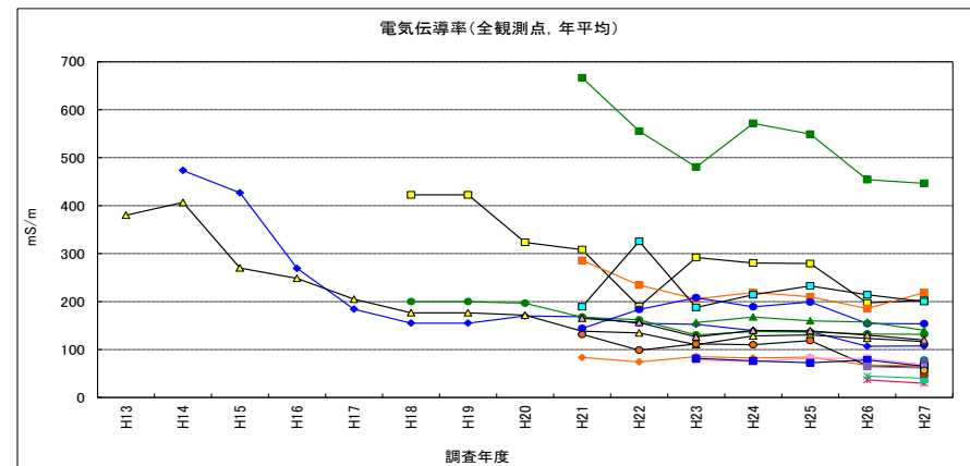
図 2-51 電気伝導率（浸透水）
