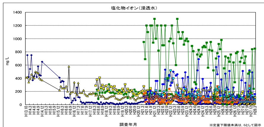
図 2-49 塩化物イオン（浸透水）
