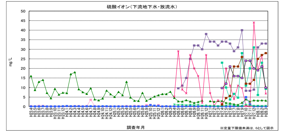
図 2-48 硫酸イオン（下流地下水、放流水）
