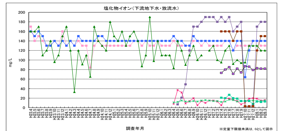
図 2-50 塩化物イオン（下流地下水、放流水）
