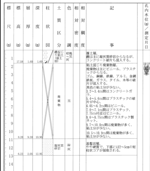
ボーリング柱状図
