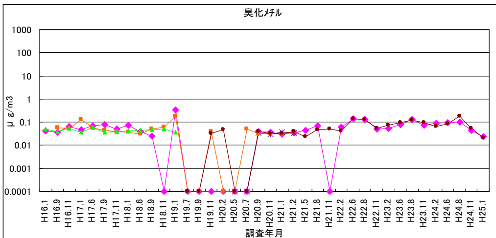
図 1-27 臭化メチル
