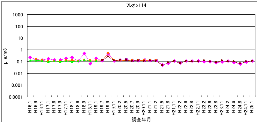
図 1-26 フレオン 114
