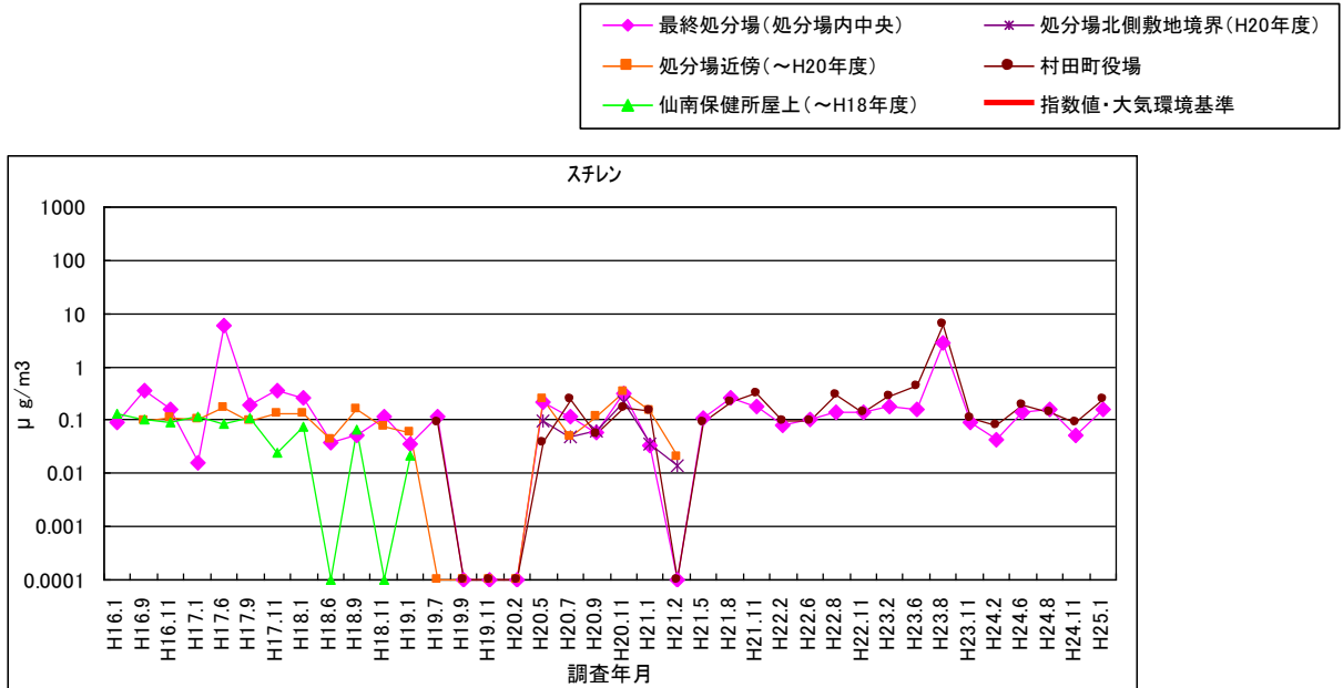
図 1-40 スチレン
