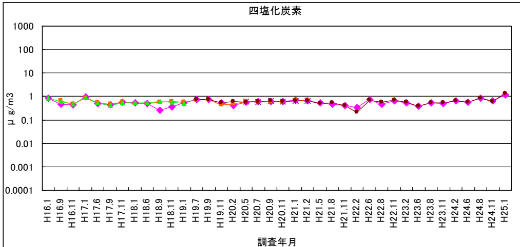
図 1-32 四塩化炭素
