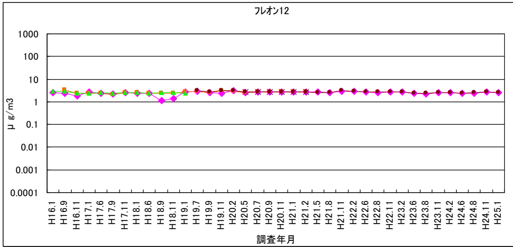
図 1-25 フレオン 12
