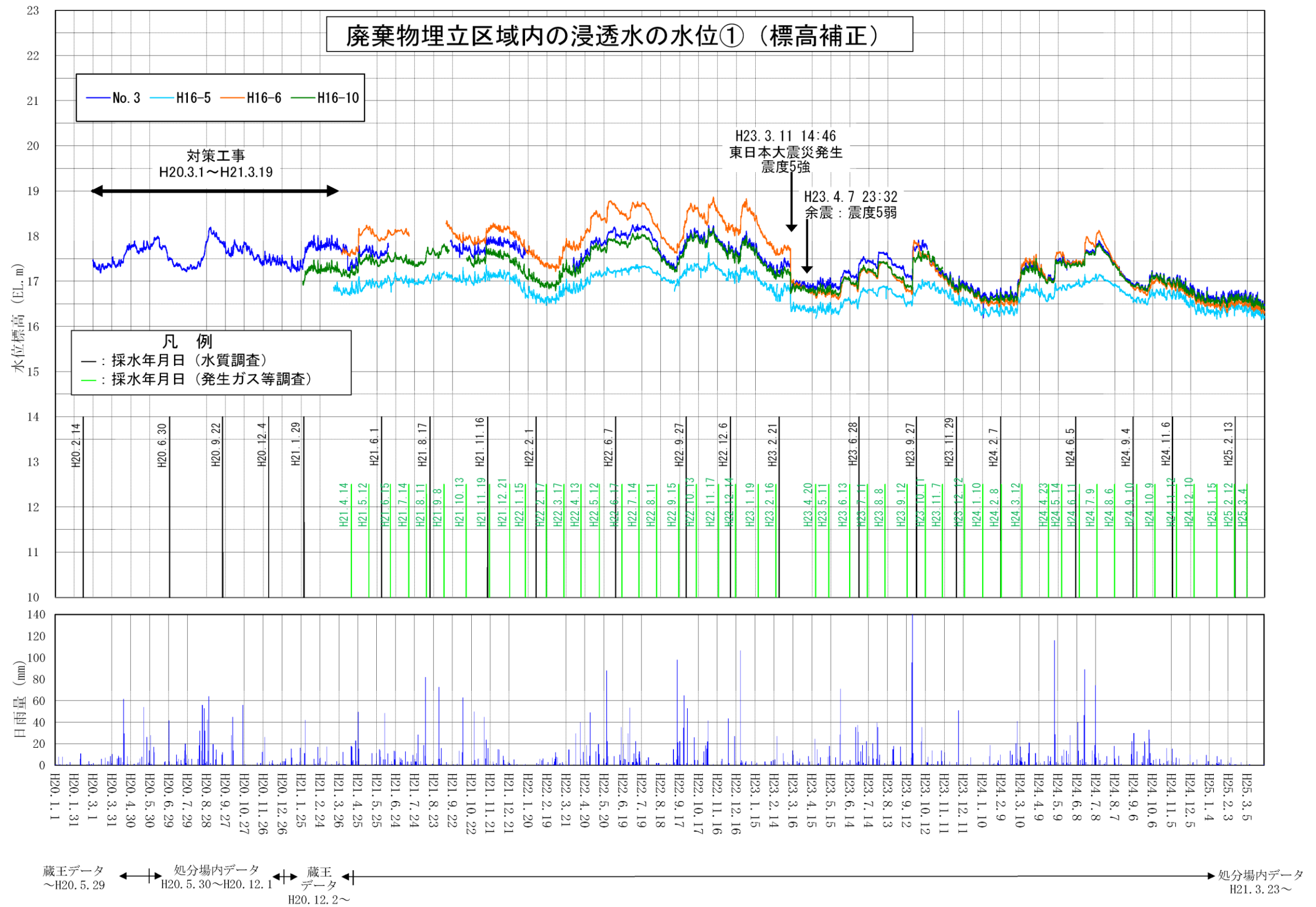
図 6-4 地下水経時変化図 (廃棄物埋立区域内の浸透水の水位①)
