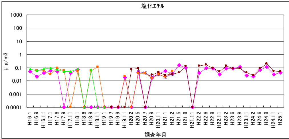
図 1-19 塩化エチル
