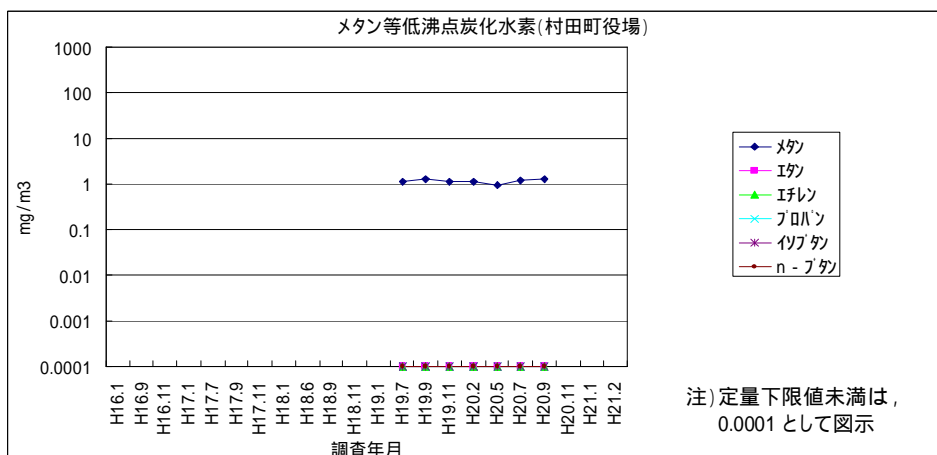
図 1-22 メタン等低沸点炭化水素(村田町役場)
