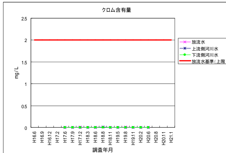
図 4-72 ク롬含有量 (放流水・河川水)
