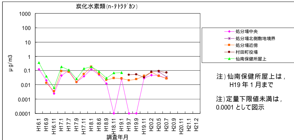
図 1-42 炭化水素類 (n-テトラデカン)
