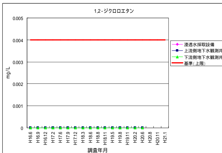
図 4-12 1,2-ジクロロエタン (浸透水・地下水)
