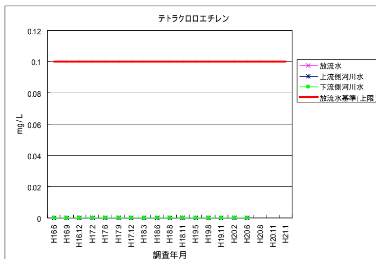
図 4-45 テトラクロロエチレン (放流水・河川水)
