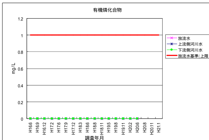
図 4-39 有機燐化合物 (放流水・河川水)
