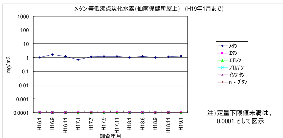
図 1-23 炭化水素等低沸点炭化水素(仙南保健所屋上)(H19年1月まで)
