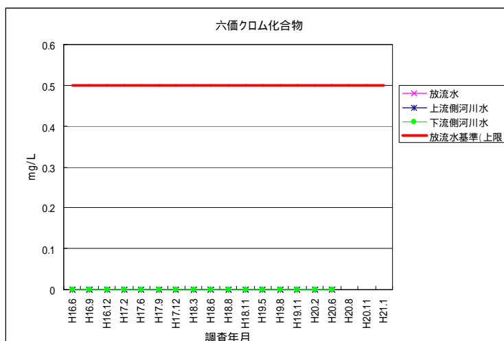
図 4-40 六価クロム化合物 (放流水・河川水)
