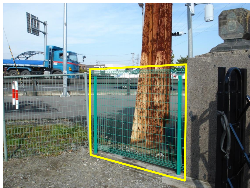
【改修後】
