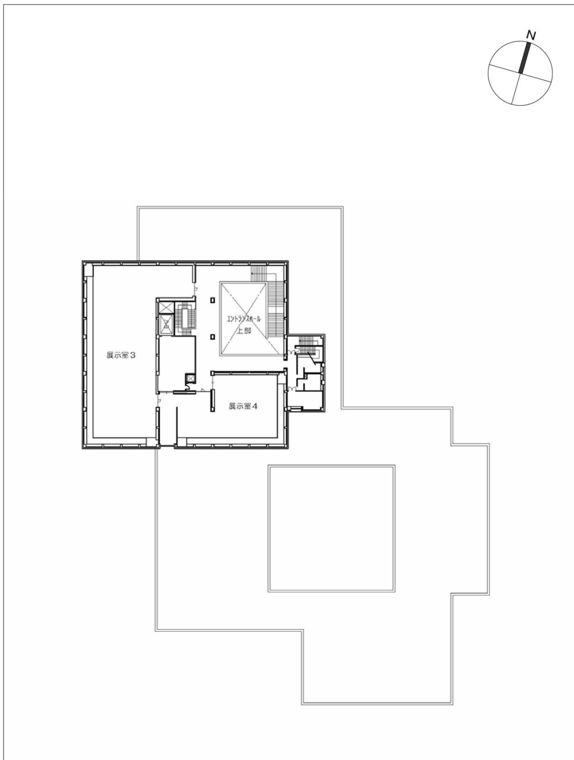
【図5】宮城県美術館の既存本館 2階平面図
