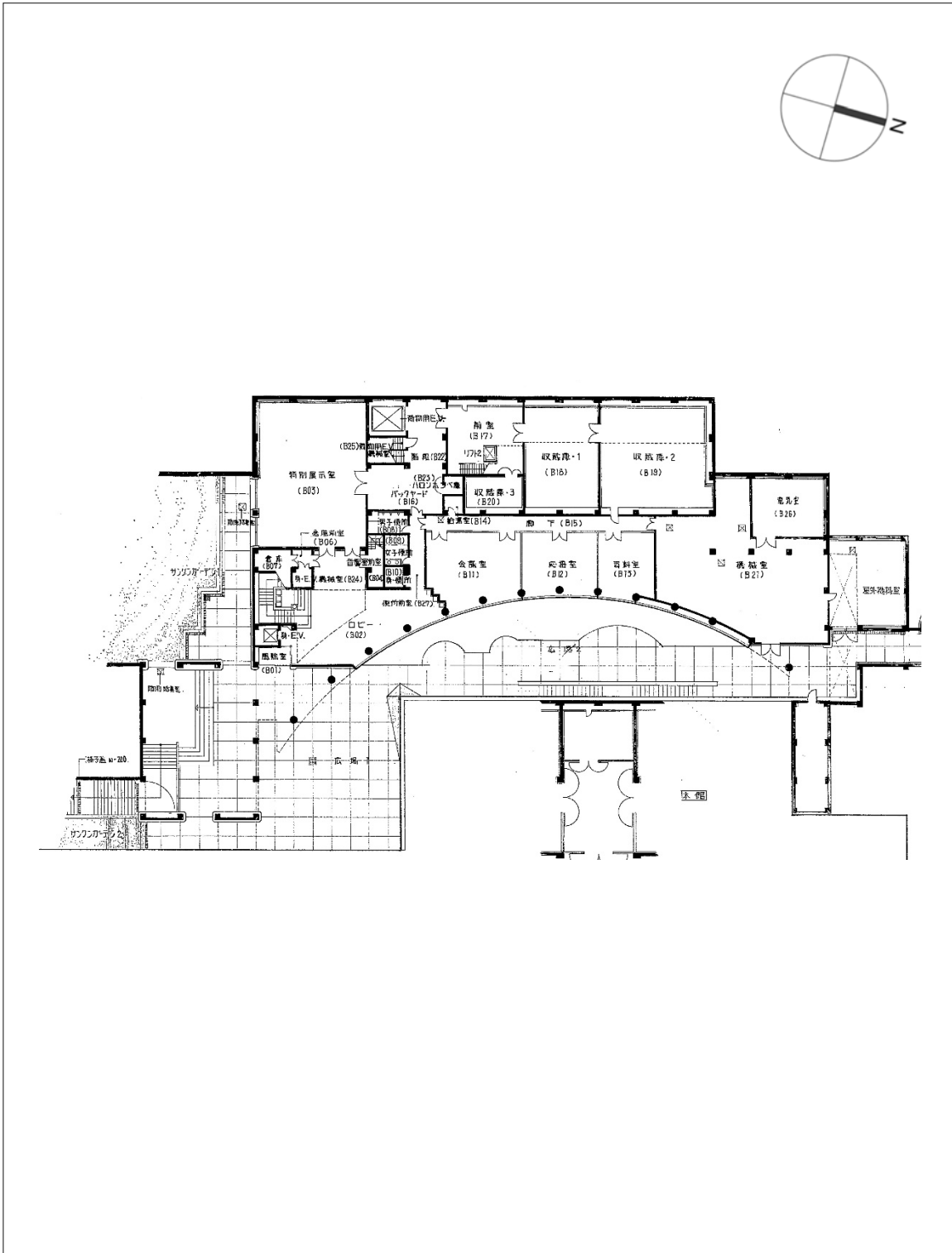
【図6】宮城県美術館の既存佐藤忠良記念館 地階平面図
