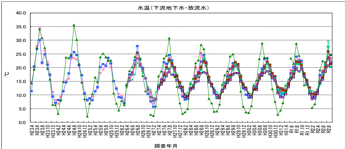
図 4-8 水温
