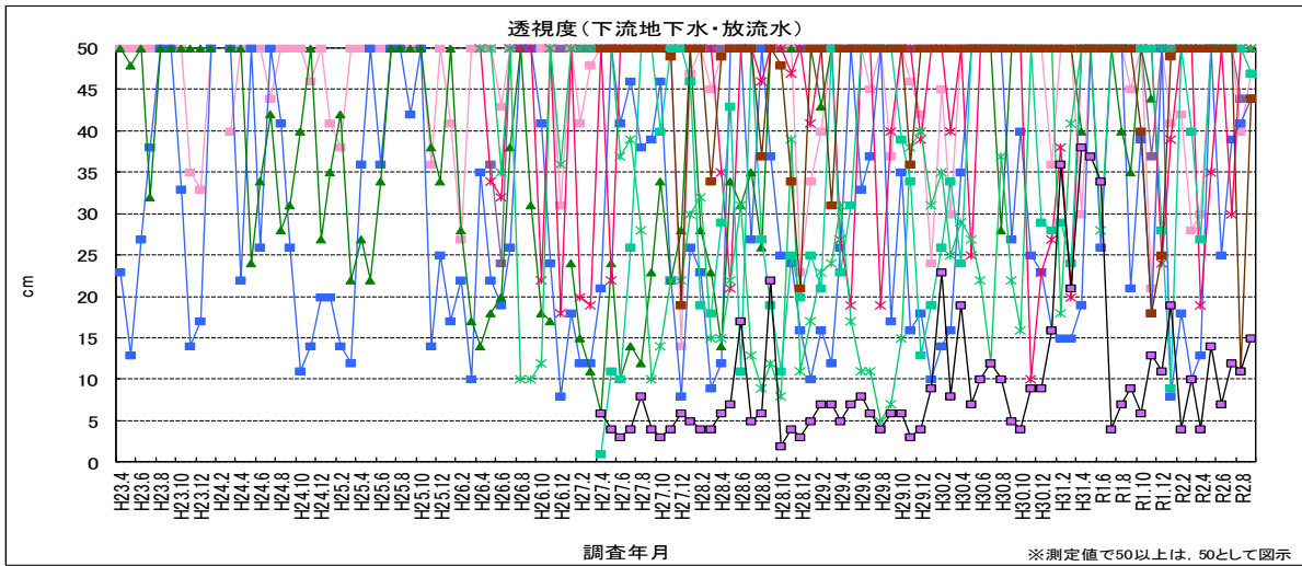
図 4-9 透視度
