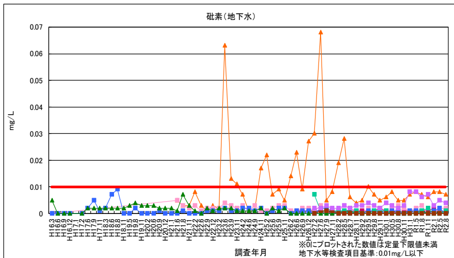
図 3-10 砒素（地下水）
