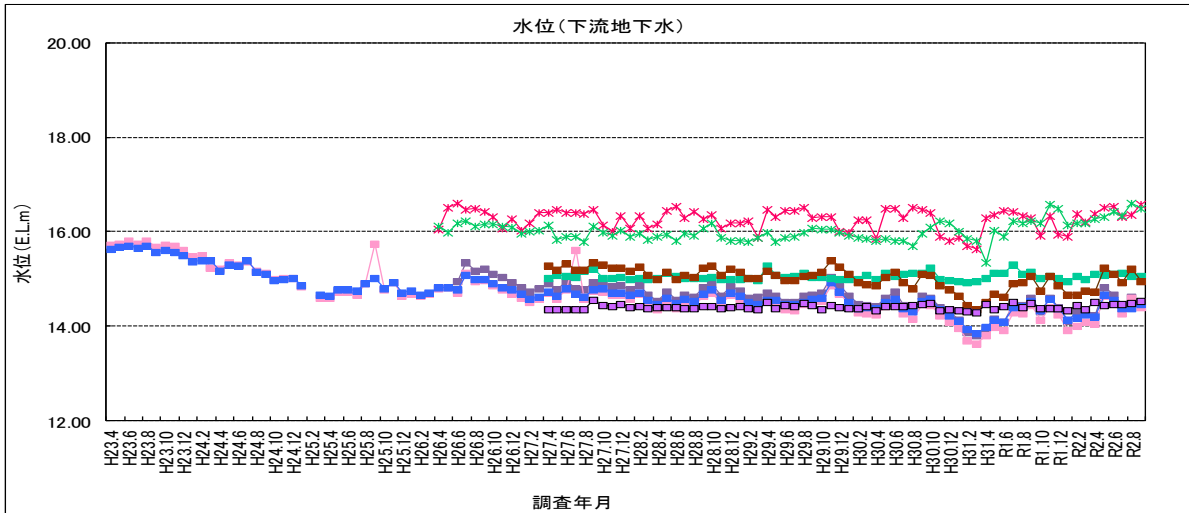
図 4-7 水位
