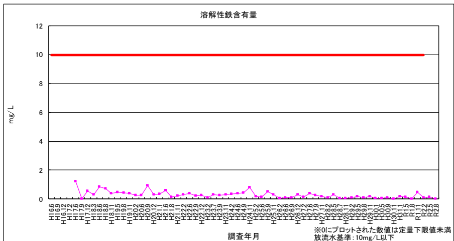
図 2-20 溶解性鉄含有量（放流水）
