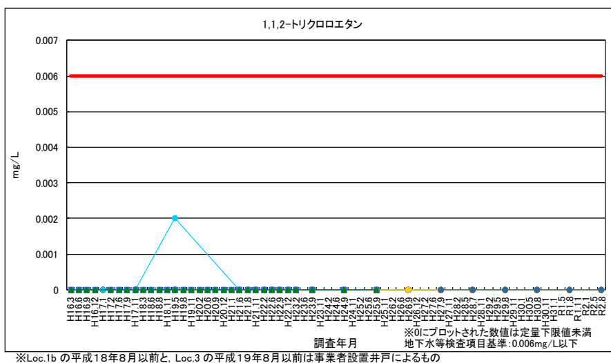
図 3-22 1,1,2-トリクロロエタン (浸透水・地下水)
