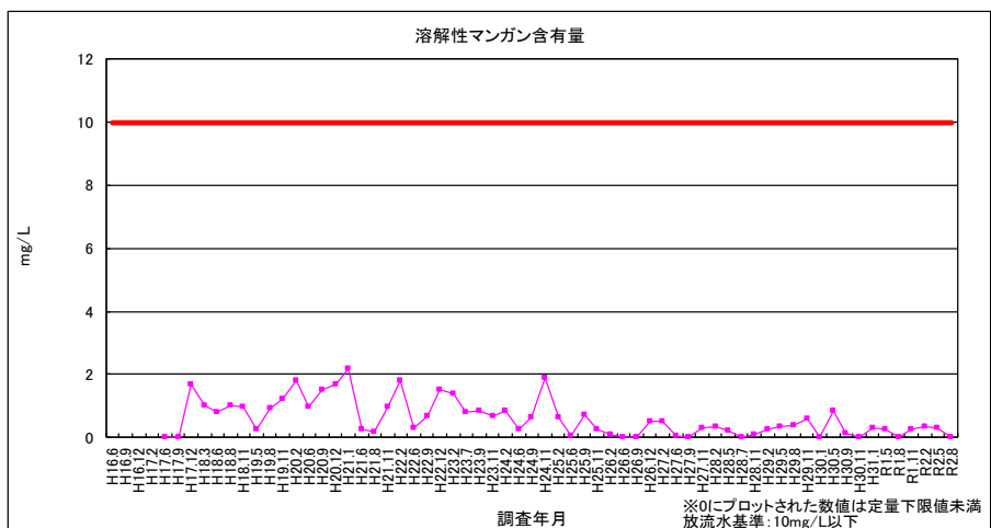
図 2-21 溶解性マンガン含有量（放流水）
