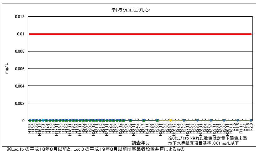
図 3-14 テトラクロロエチレン (浸透水・地下水)
