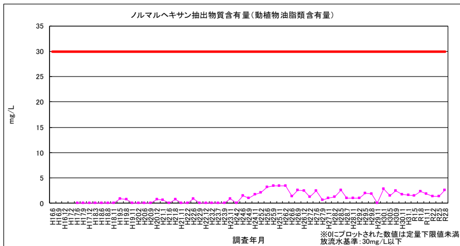
図 2-16 ノルマルヘキサン抽出物質含有量（動植物油脂類含有量）（放流水）
