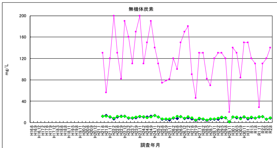
図 2-25 無機体炭素（放流水・河川水）
