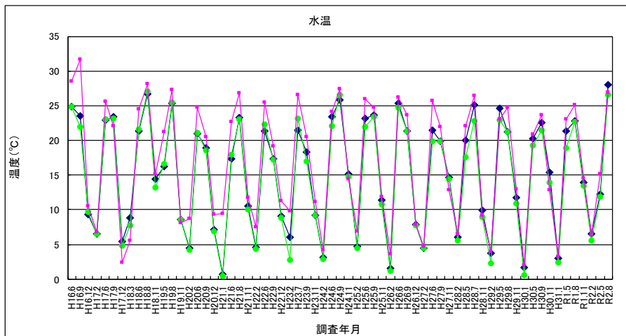
図 2-28 水温（放流水・河川水）
