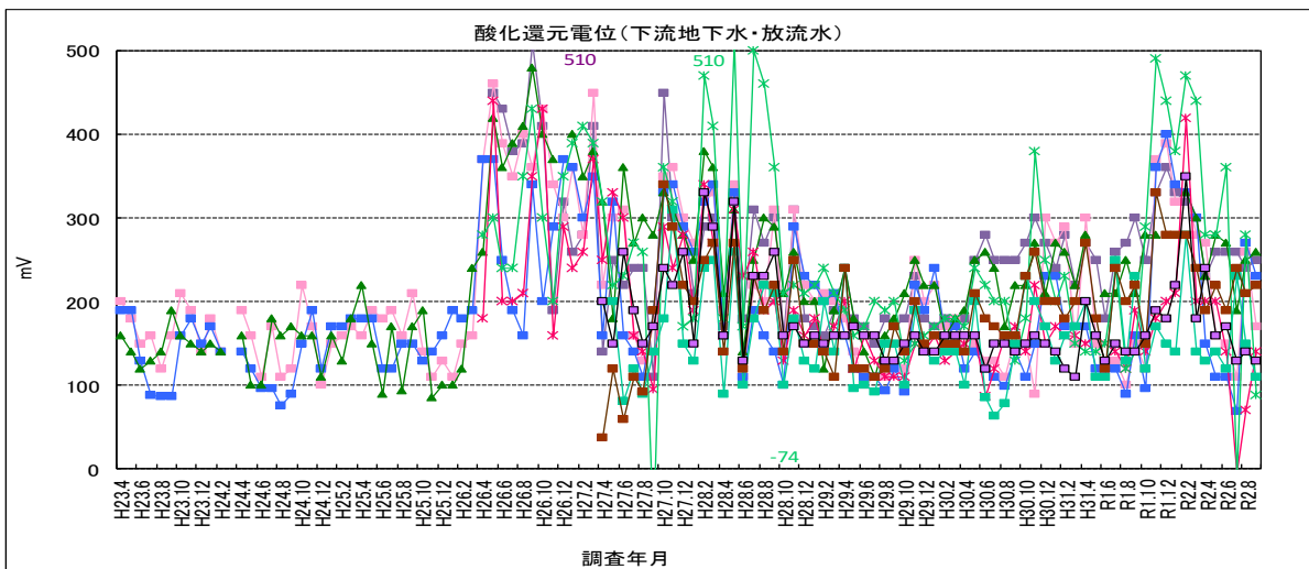
図 4-14 酸化還元電位
