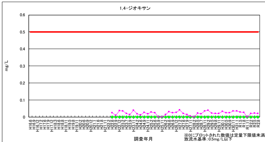
図 2-8 1,4-ジオキサン（放流水・河川水）
