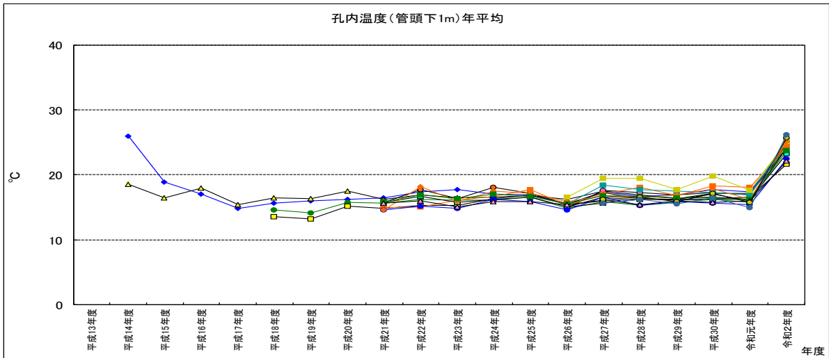
図 4-6 孔内温度（管頭下 1m で測定）
