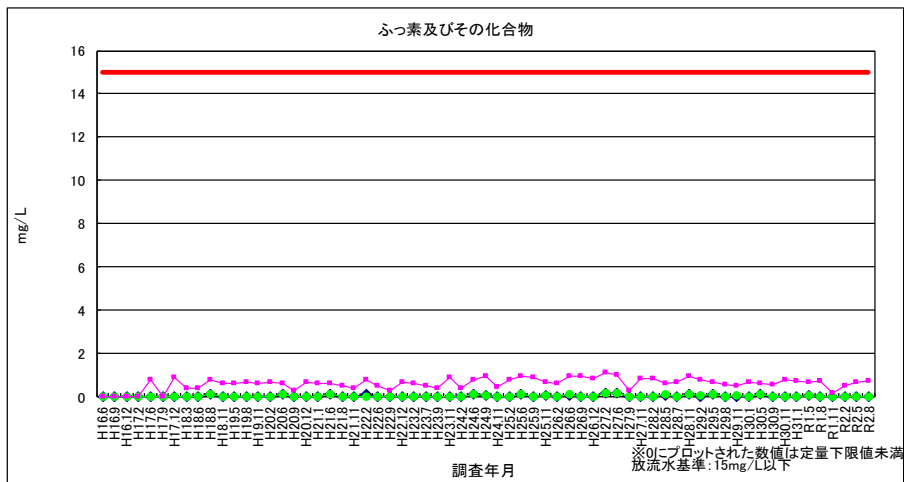
図 2-10 ふっ素及びその化合物（放流水・河川水）
