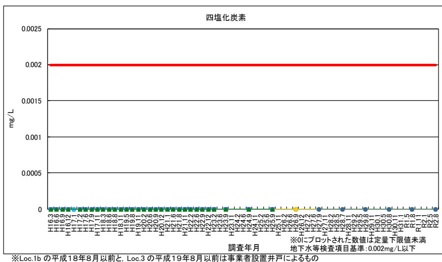
図 3-16 四塩化炭素（浸透水・地下水）
