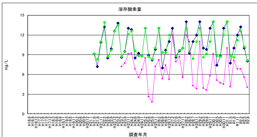
図 2-24 溶存酸素量（河川水・放流水）
