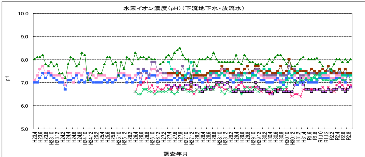
図 4-10 水素イオン濃度 (pH)
