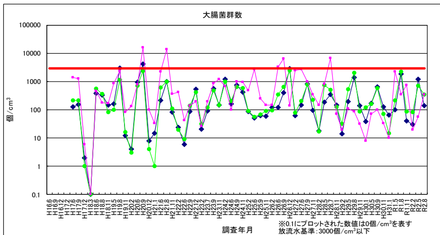
図 2-23 大腸菌群数（放流水・河川水）
