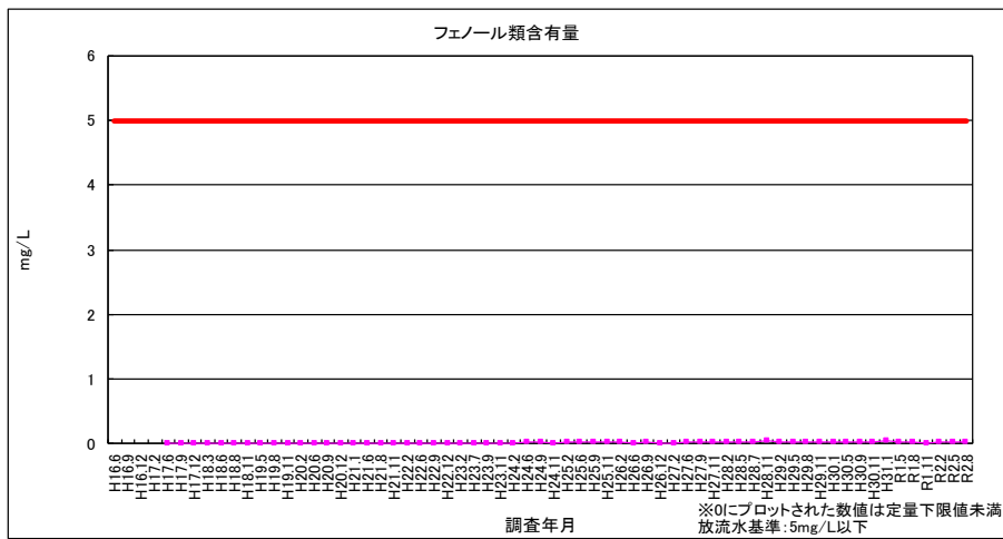
図 2-17 フェノール類含有量（放流水）
