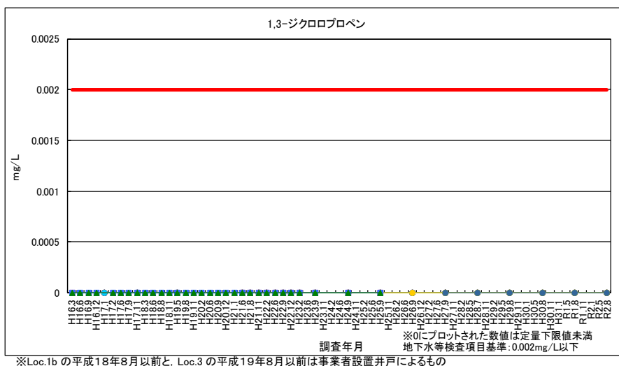
図 3-23 1,3-ジクロロプロペン (浸透水・地下水)
