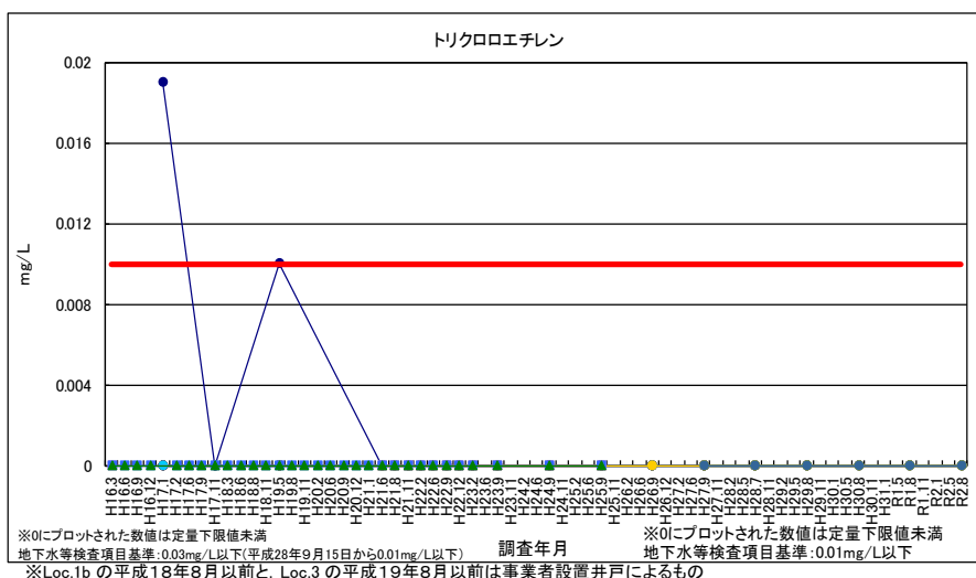
図 3-13 トリクロロエチレン (浸透水・地下水)
