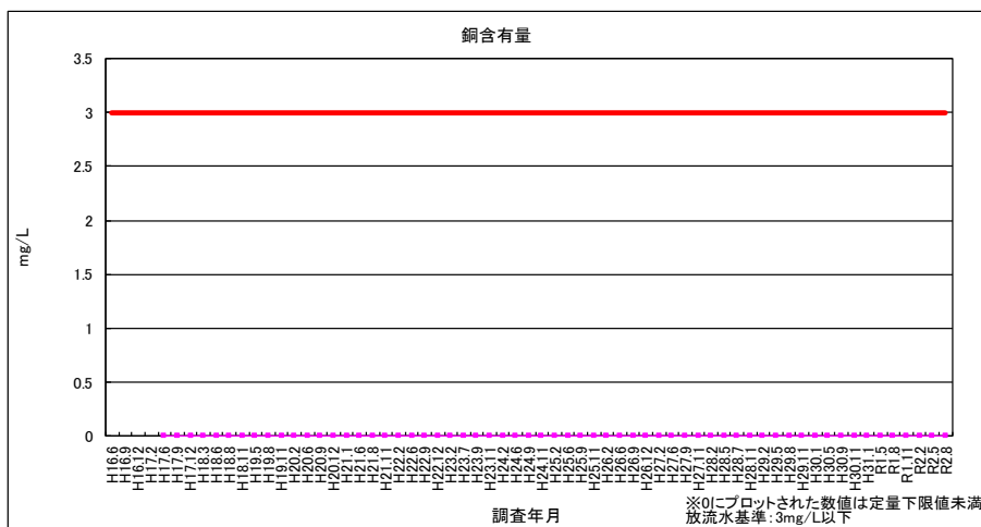
図 2-18 銅含有量（放流水）
