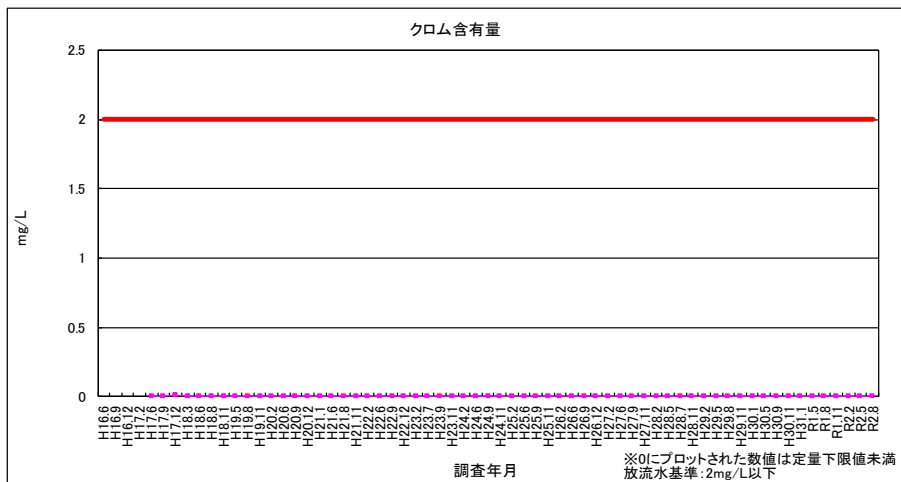
図 2-22 クロム含有量（放流水）
