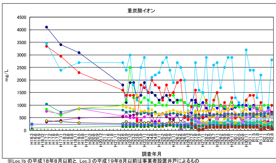
図 3-47 重炭酸イオン（浸透水・地下水）
