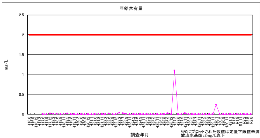
図 2-19 亜鉛含有量（放流水）
