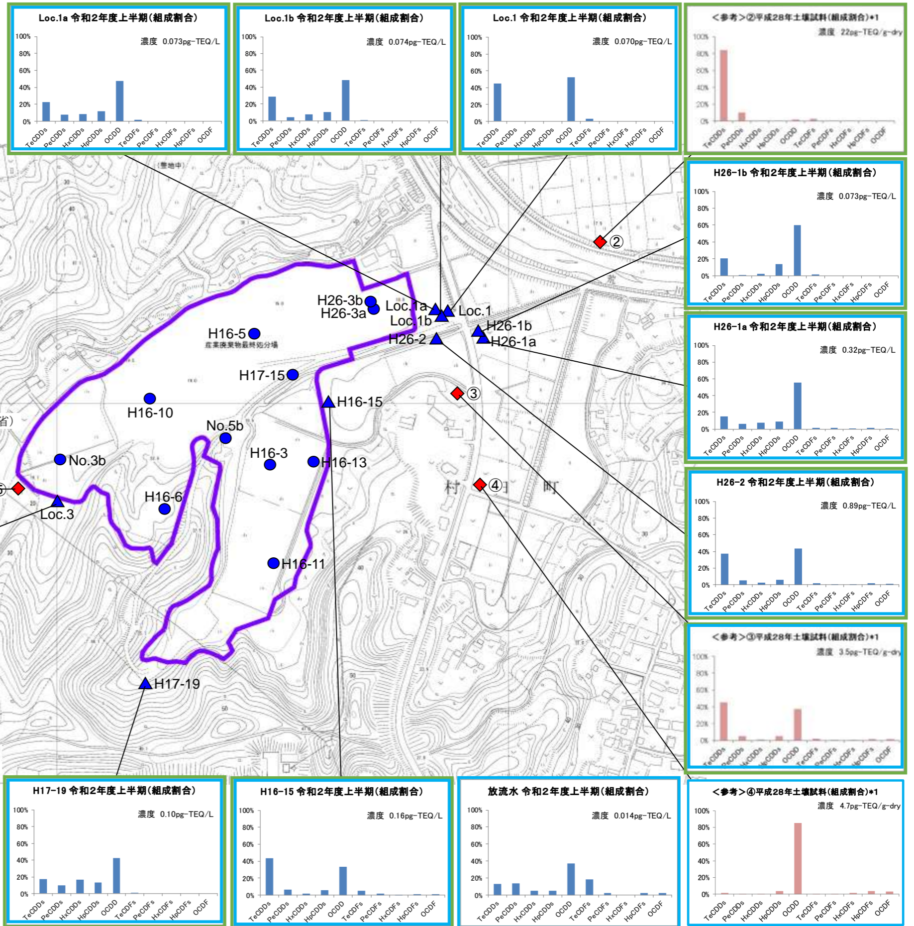
図3-2 ダイオキシン類パターン (令和2年度上半期・処分場外)
