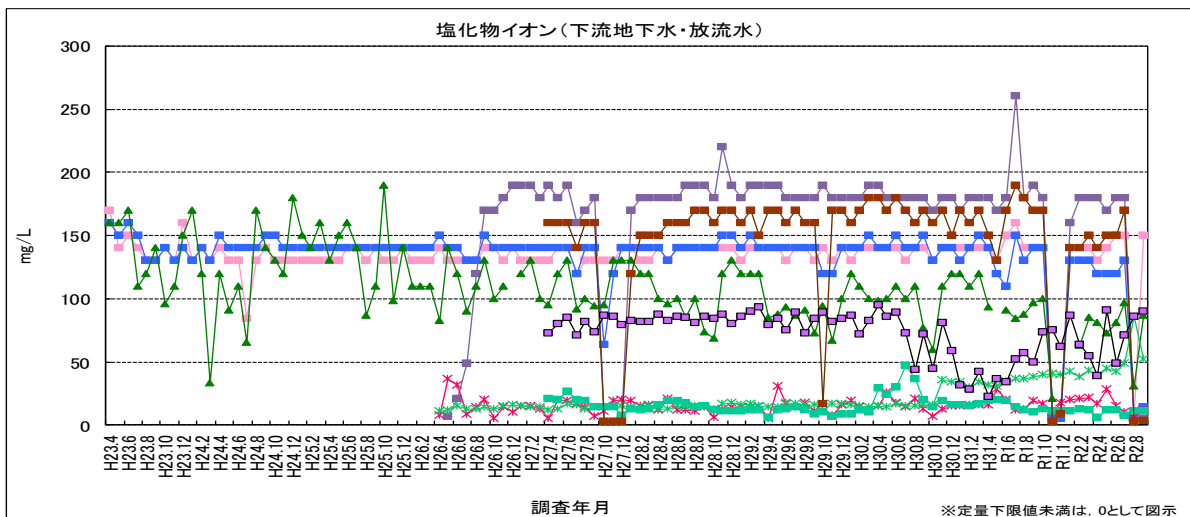
図 4-12 塩化物イオン
