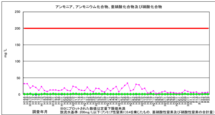
図 2-11 アンモニア、アンモニウム化合物、亜硝酸化合物及び硝酸化合物（放流水・河川水）
