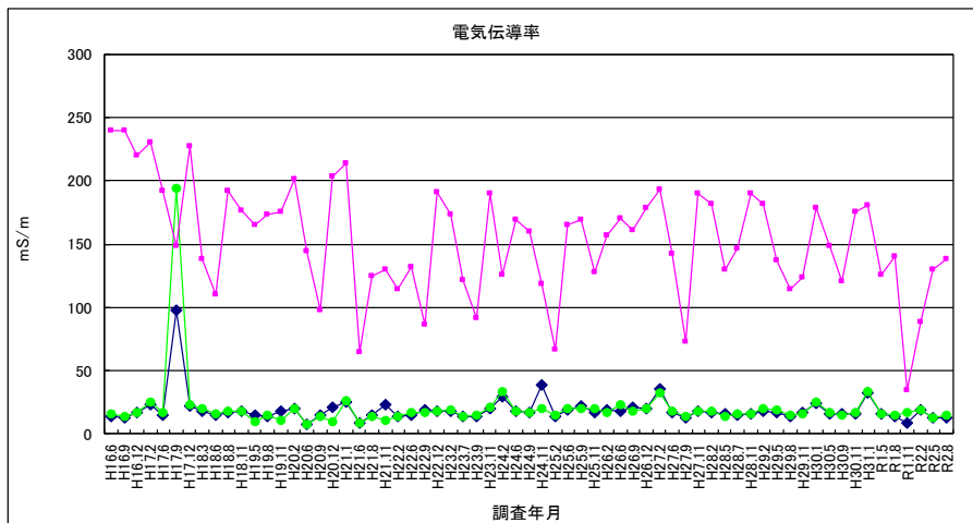
図 2-31 電気伝導率（放流水・河川水）
