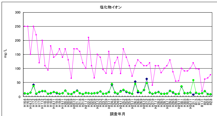
図 2-26 塩化物イオン（放流水・河川水）
