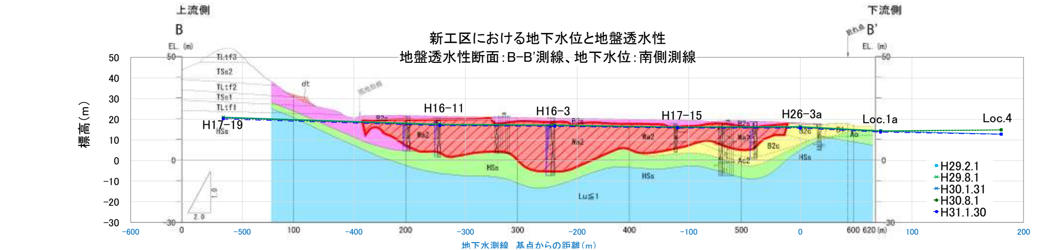
図 2-59 平成30年度下期の上流側～下流側にかけての水位標高変化（地盤透水性断面図）
