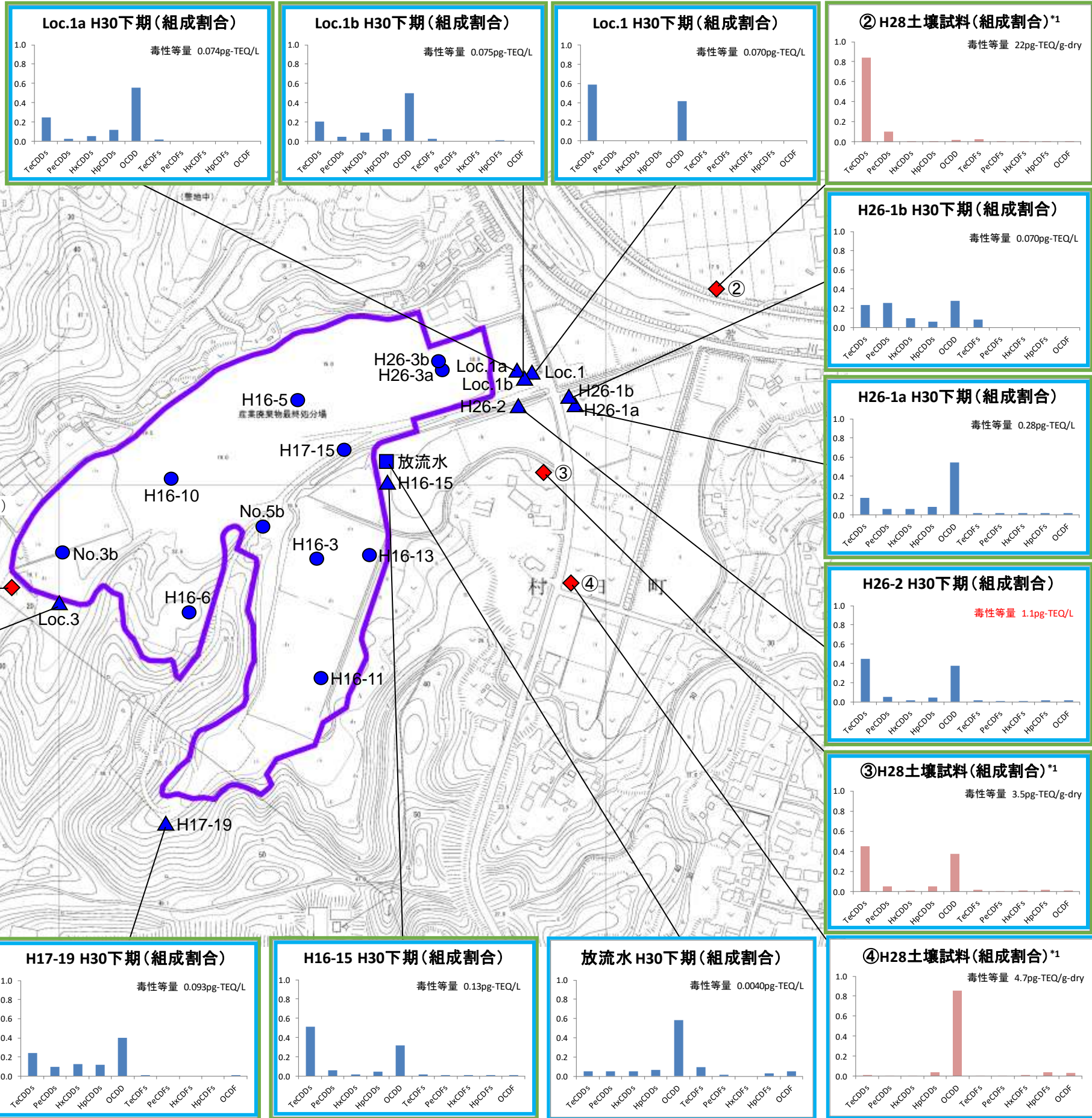
図 2-45 ダイオキシン類パターン (H30 下期・処分場外)
