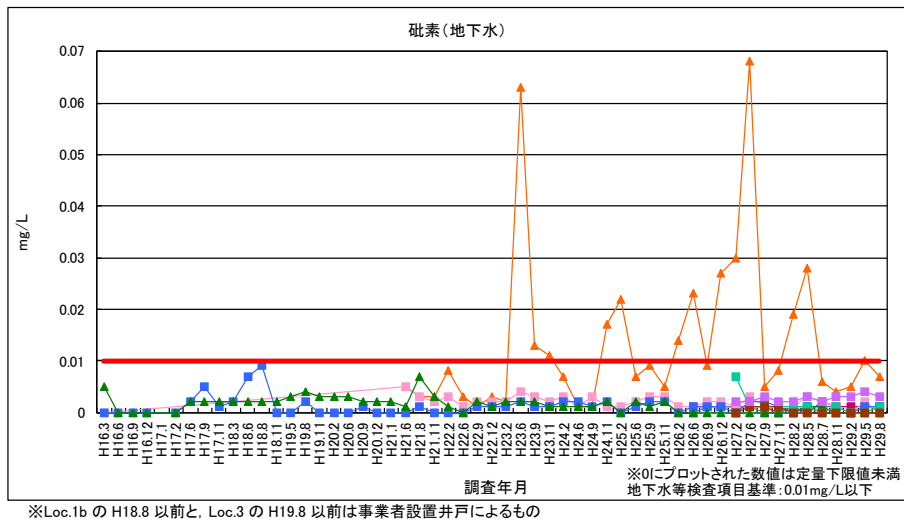
図 3-10 砒素 (地下水)
