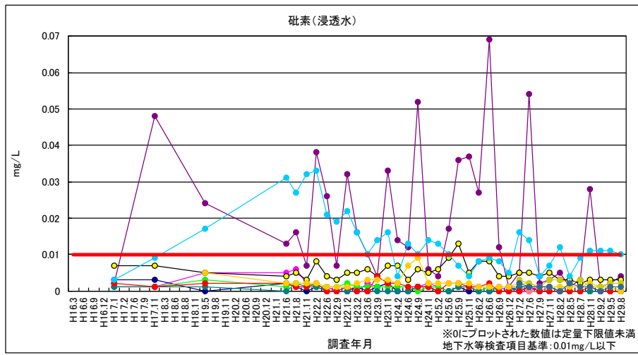
図 3-9 砒素 (浸透水)
