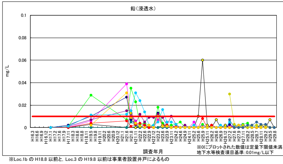
図 3-6 鉛 (浸透水)
