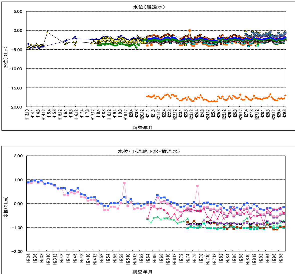
図 4-7 水位
