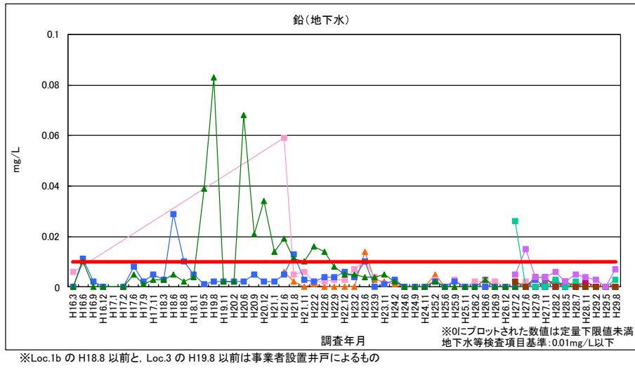
図 3-7 鉛 (地下水)
