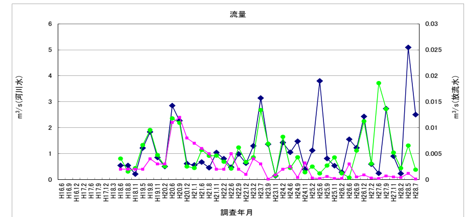
図 2-23 流量
