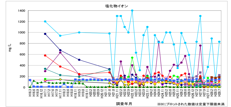
図 2-41 塩化物イオン
