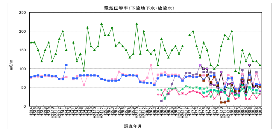
図 2-54 電気伝導率（下流地下水、放流水）
