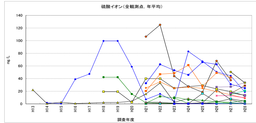
図 2-49 硫酸イオン（浸透水）
