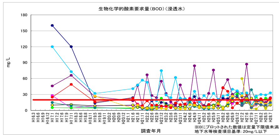
図 2-33 生物学的酸素要求量（BOD）（浸透水）
