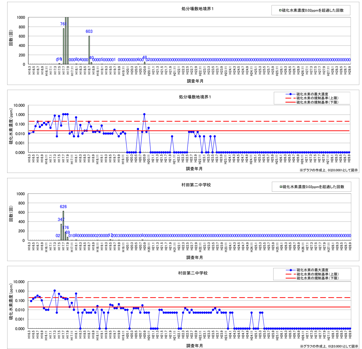
図 2-16 硫化水素連続調査結果図
