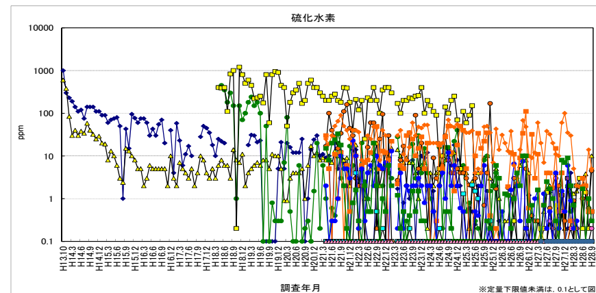
図 2-45 硫化水素 (管頭下 1m で測定) ※下図：対数表示
