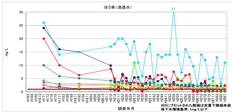
図 2-36 ほう素（浸透水）
