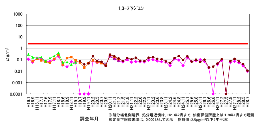
図 2-10 1,3-ブタジエン
