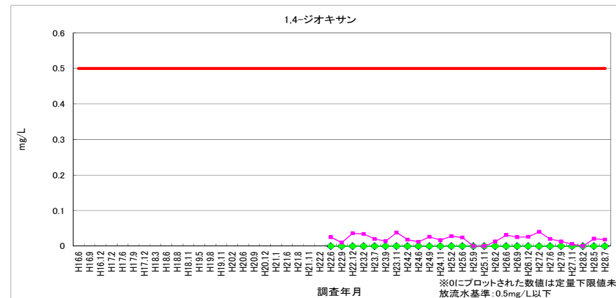
図 2-22 1,4-ジオキサン
