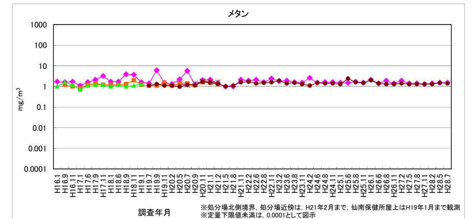
図 2-12 メタン
