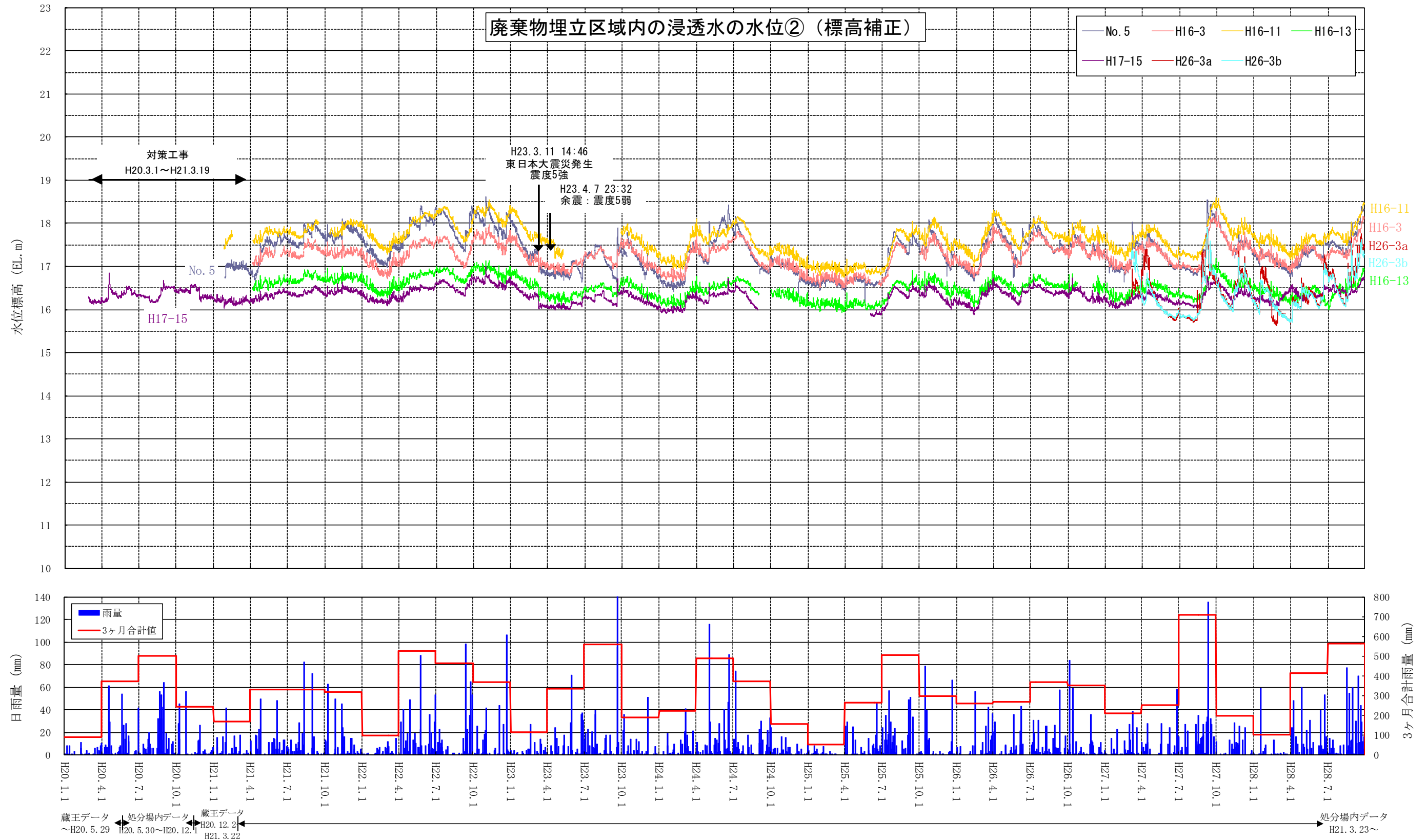
図 2-62 地下水水位経時変化図 (廃棄物埋立区域内の浸透水の水位②)
