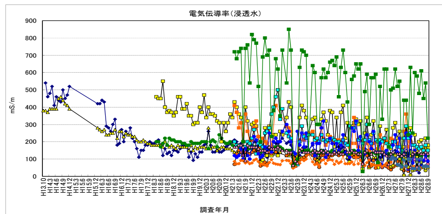
図 2-53 電気伝導率（浸透水）
