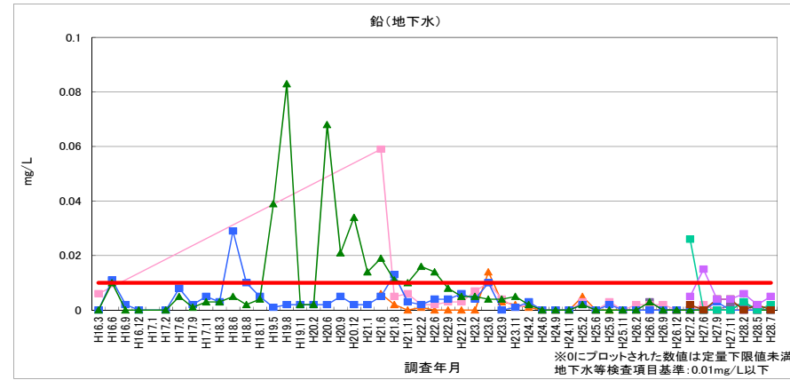
図 2-25 鉛（地下水）
