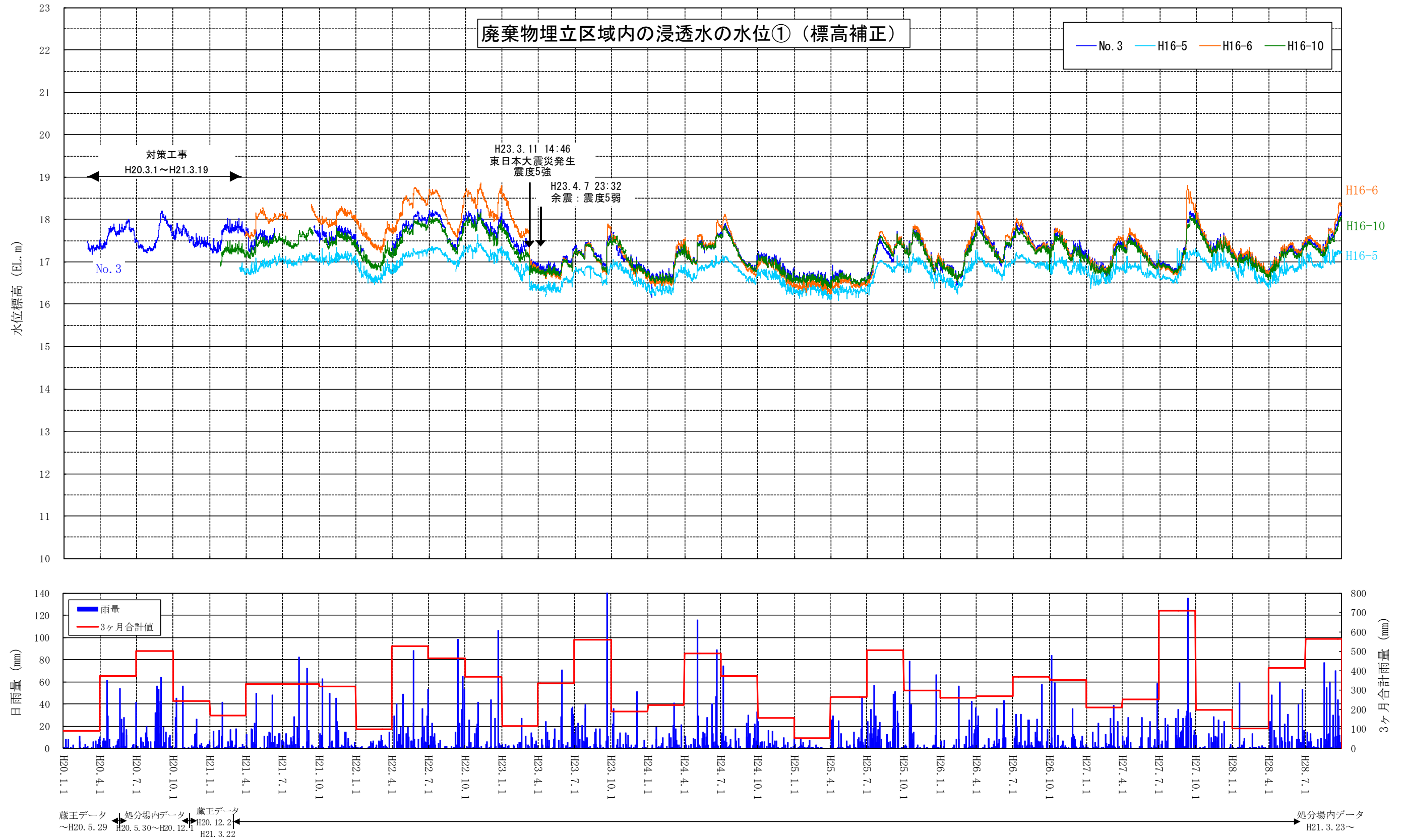
図 2-61 地下水水位経時変化図 (廃棄物埋立区域内の浸透水の水位①)
