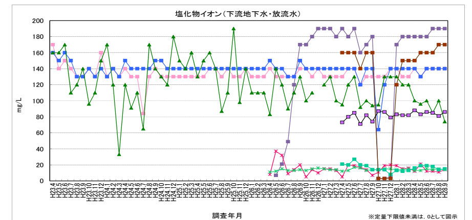
図 2-52 塩化物イオン（下流地下水、放流水）
