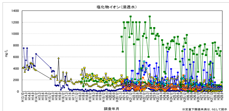
図 2-51 塩化物イオン（浸透水）
