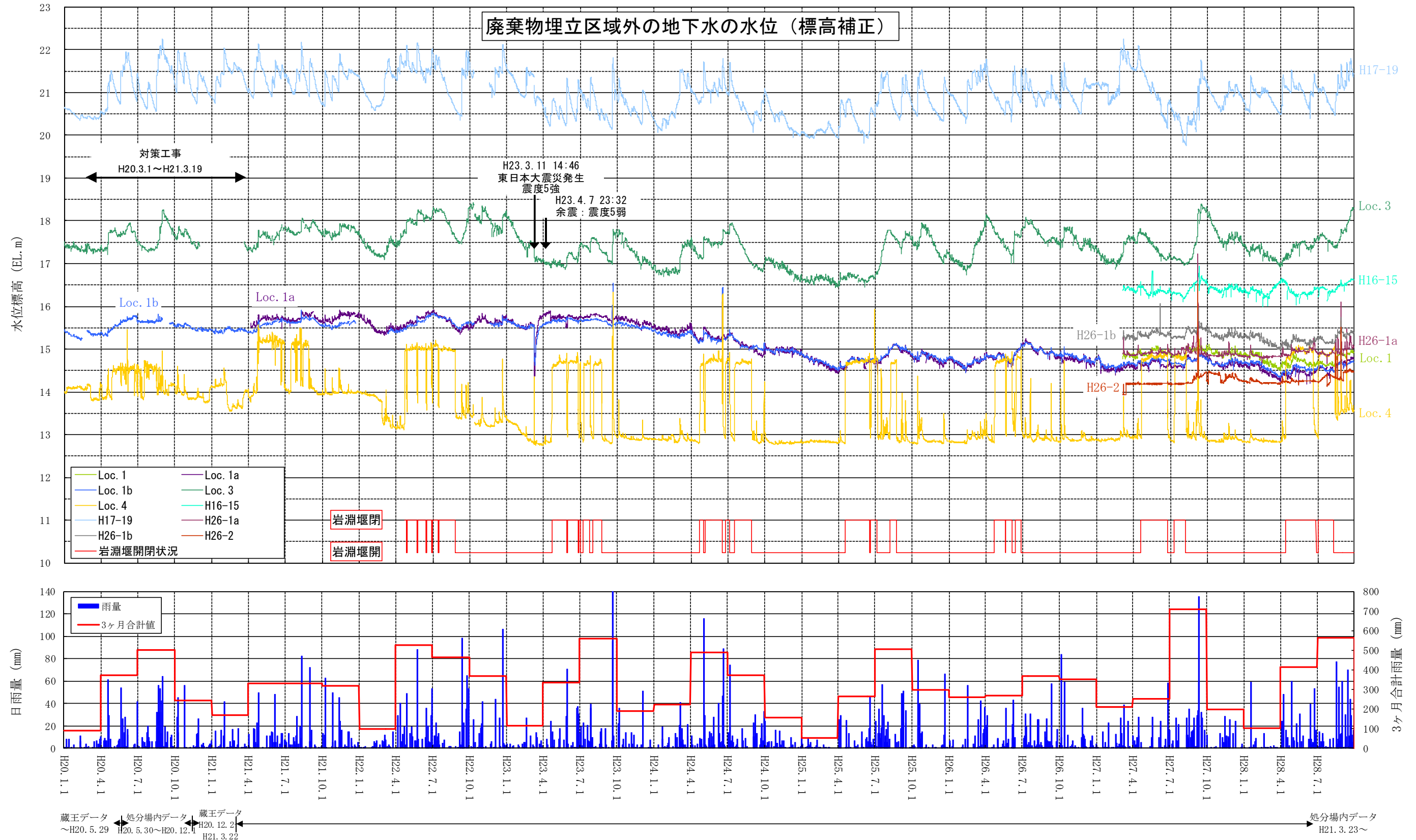
図 2-60 地下水位経時変化図（廃棄物埋立区域外の地下水の水位）
