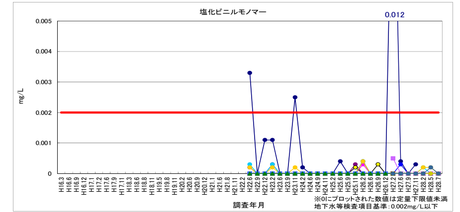
図 2-32 塩化ビニルモノマー
