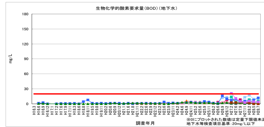
図 2-34 生物学的酸素要求量（BOD）（地下水）
