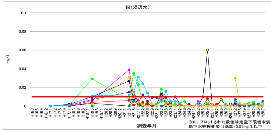
図 2-24 鉛（浸透水）
