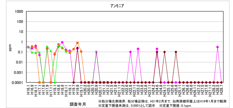
図 2-9 アンモニア
