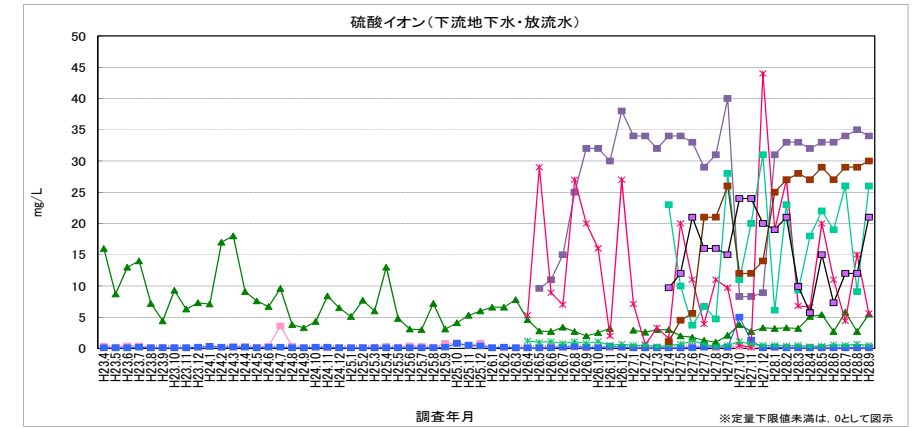
図 2-50 硫酸イオン（下流地下水、放流水）
