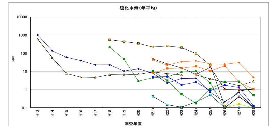
図 2-45 硫化水素 (管頭下 1m で測定) ※下図：対数表示
