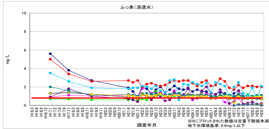
図 2-39 ふっ素 (浸透水)
