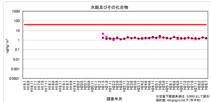
図 2-14 水銀及びその化合物
