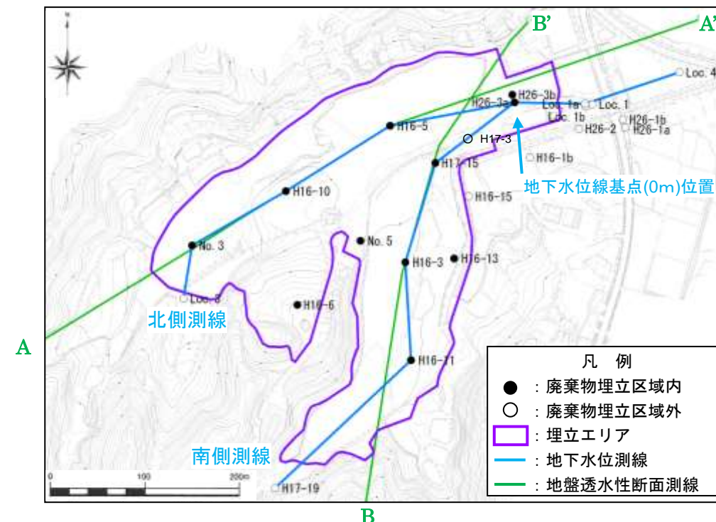
図 2-62 令和3年度上半期のの上流側～下流側にかけての水位標高変化（平面図）
