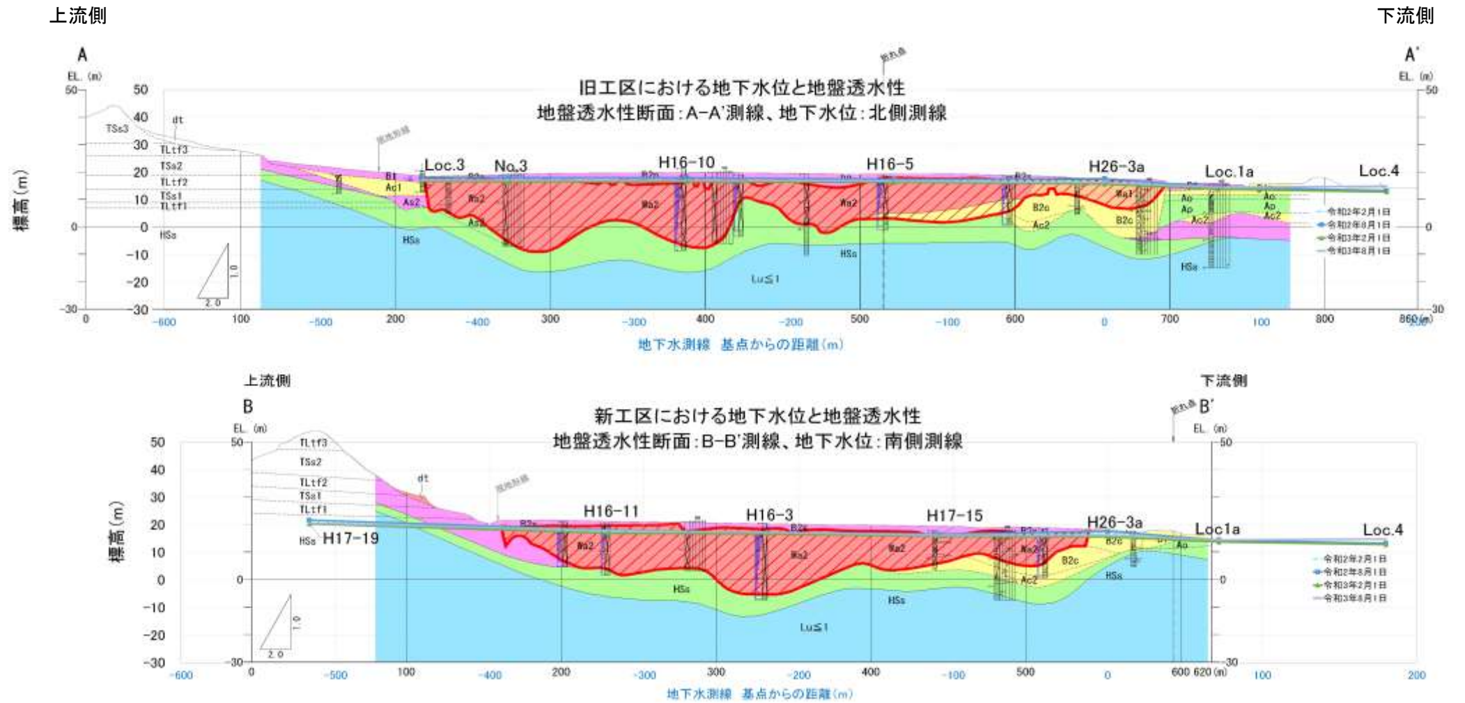
図 2-61 令和3年度上半期のの上流側～下流側にかけての水位標高変化（地盤透水性断面図）
