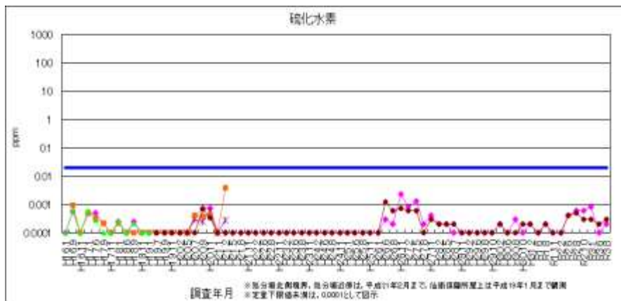
図 2-11 硫化水素
