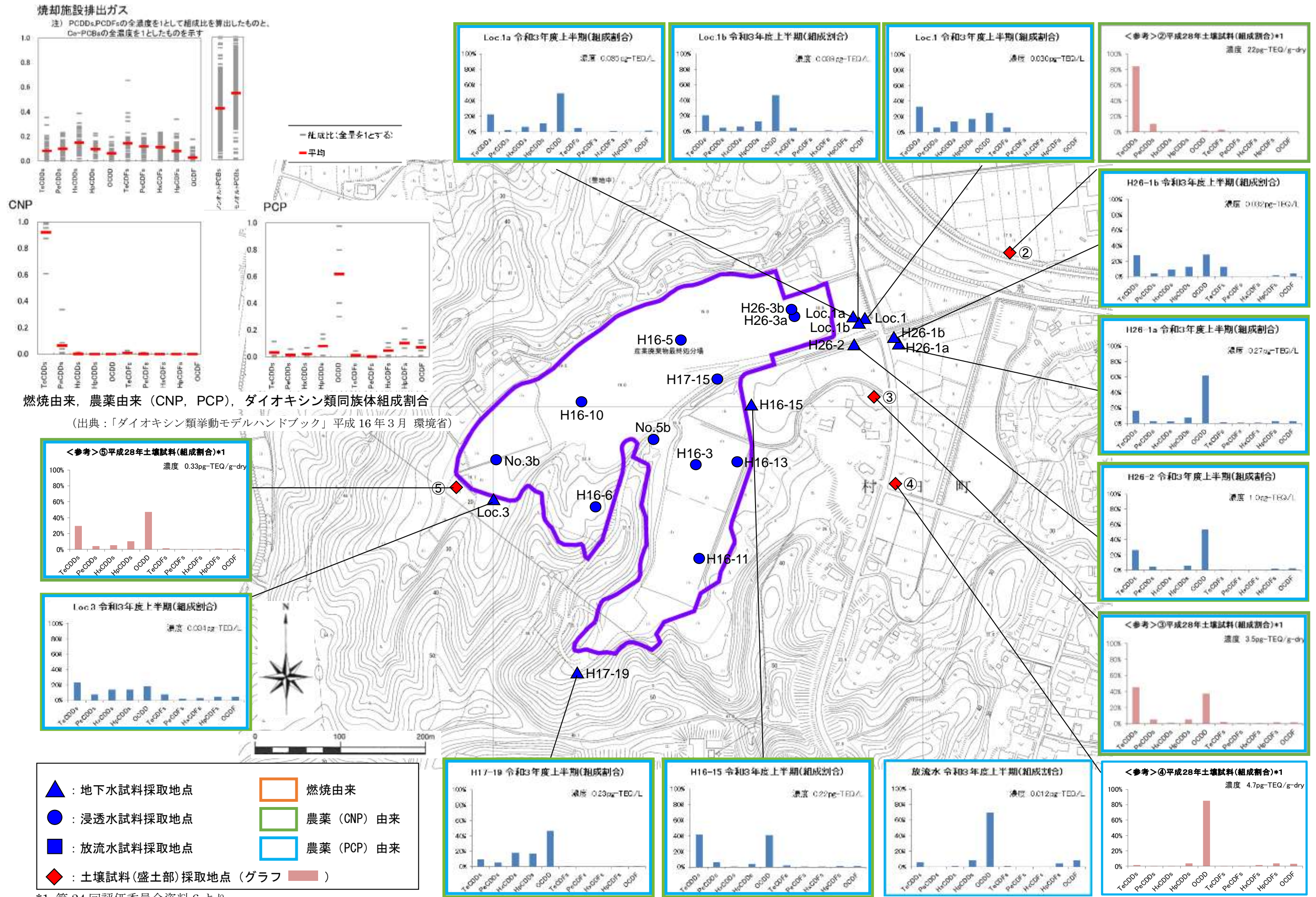
図2-47 ダイオキシン類パターン (令和3年度上半期・処分場外)
