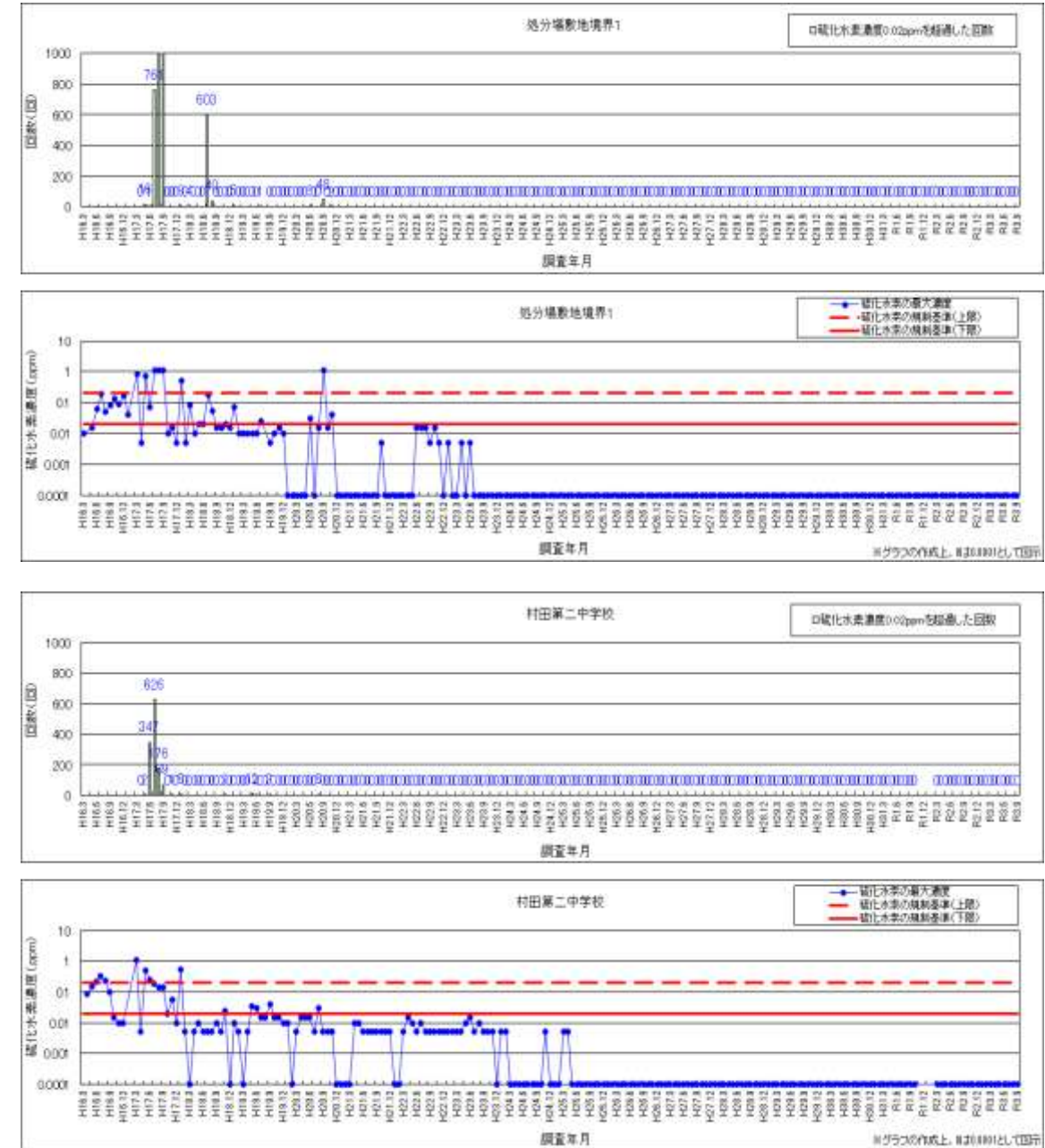
図 2-15 硫化水素連続調査結果図
