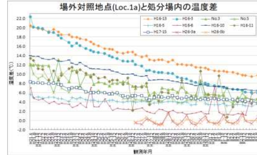
図 2-58 処分場内高温部と対照地点 (Loc.1a) との温度差の変化
