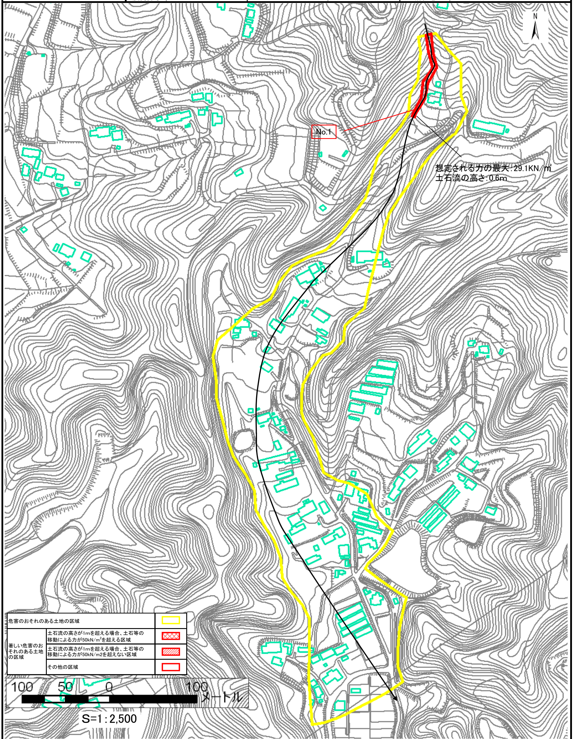
様式3-1 危害のおそれのある土地、著しい危害のおそれのある土地の設定図
