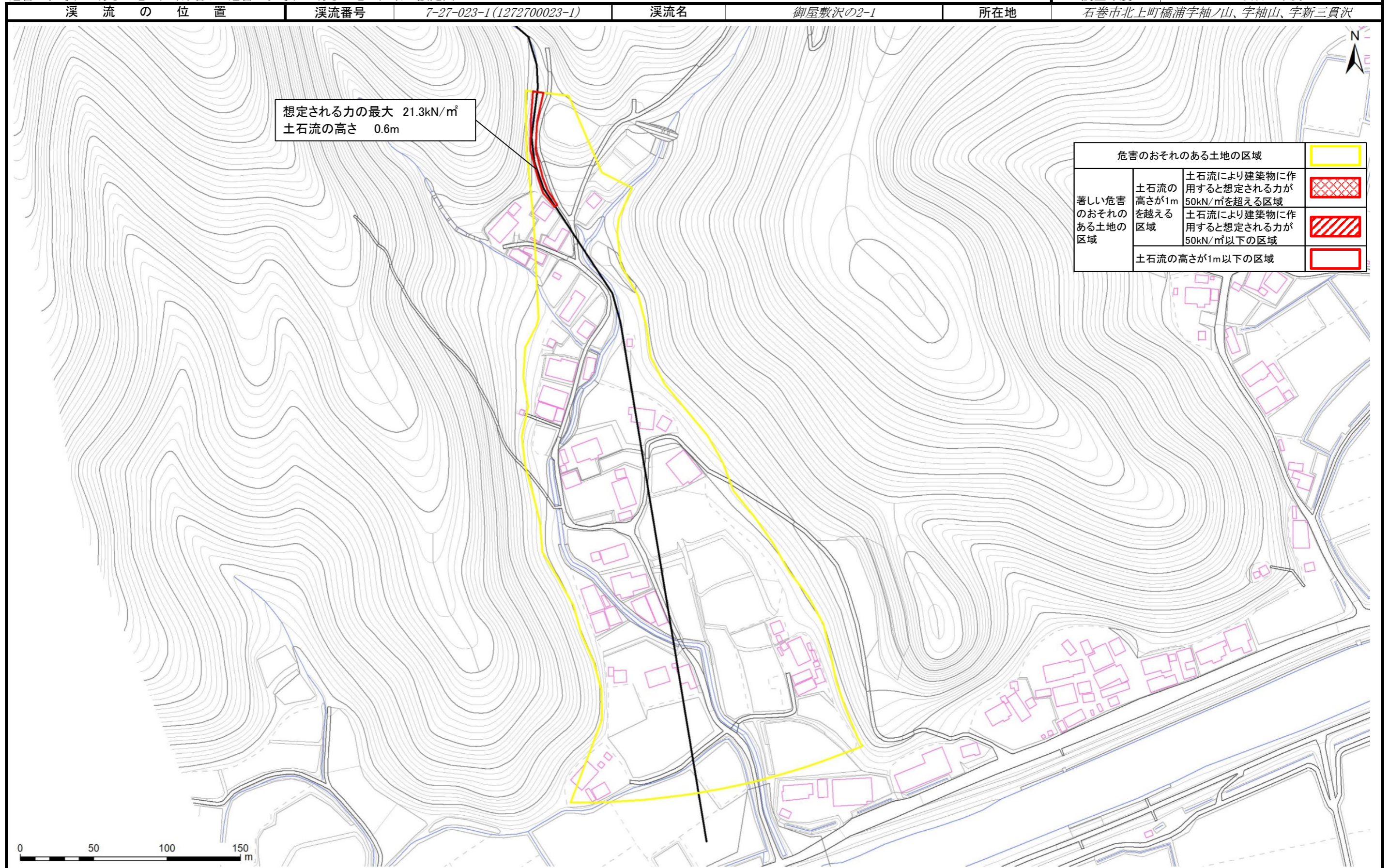
危険のおそれのある土地の区域、著しい危険のおそれのある土地の区域の設定図
