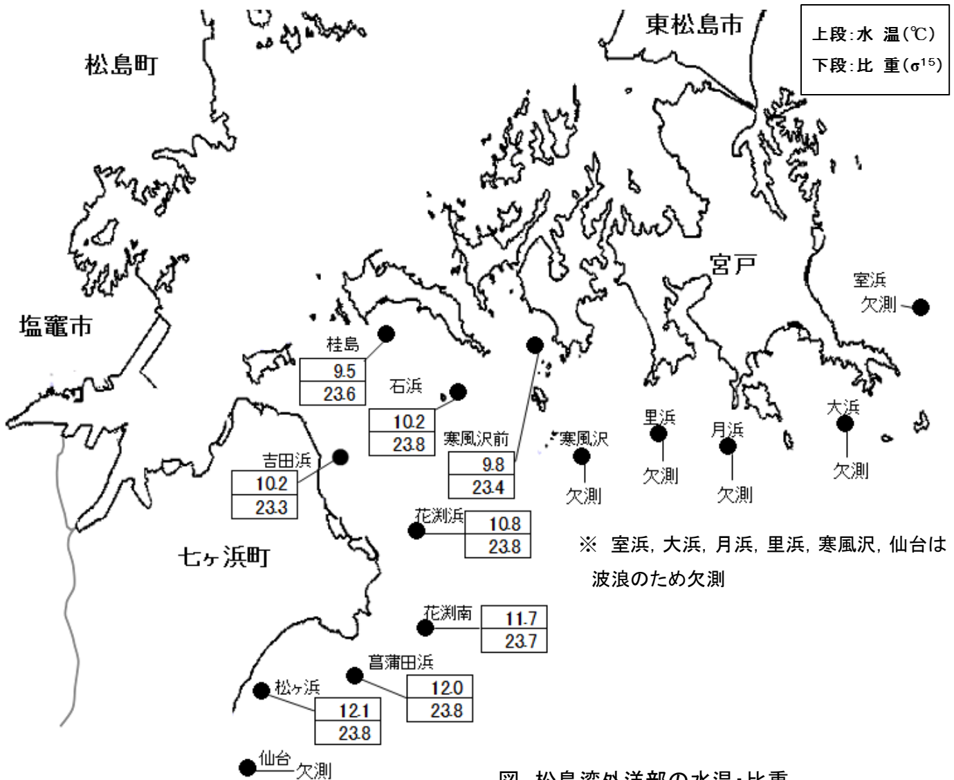
図 松島湾外洋部の水温・比重
