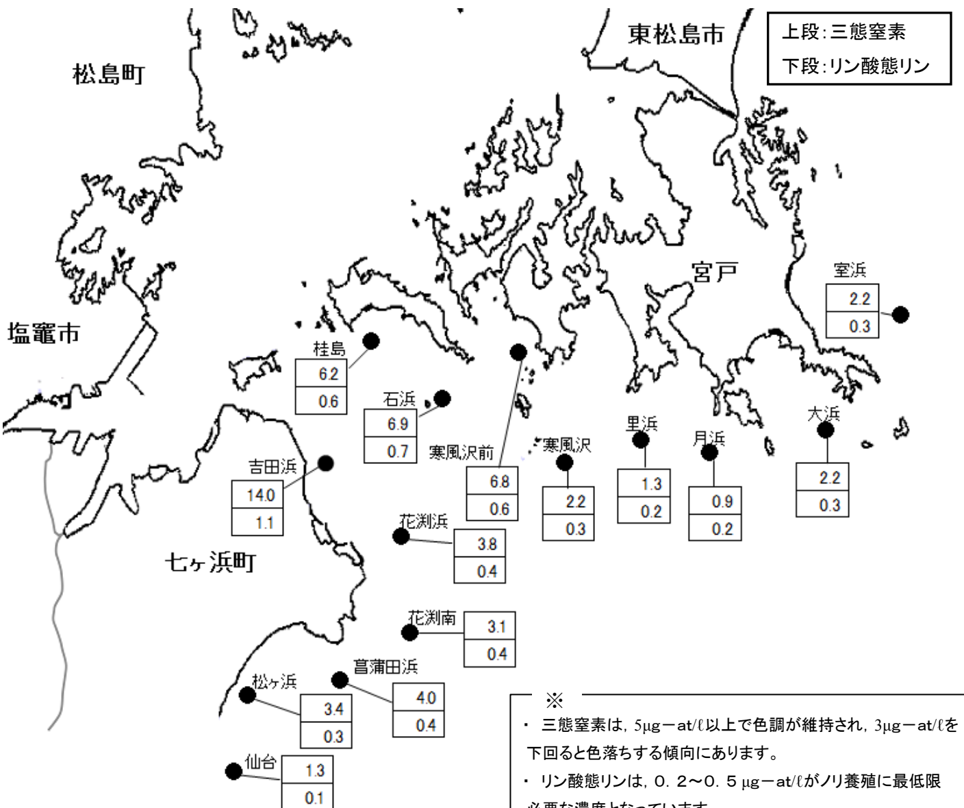
図 松島湾外洋部の栄養塩
