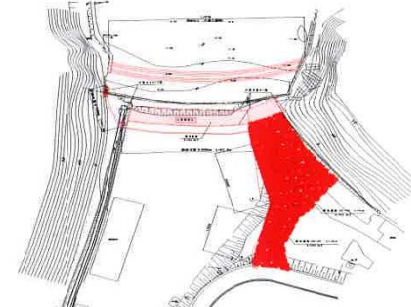
既設堤防復旧工平面図
