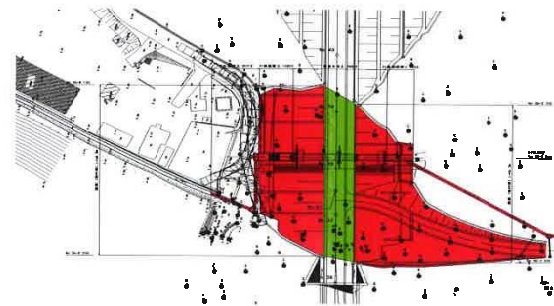
防潮堤復旧工(平面図)
