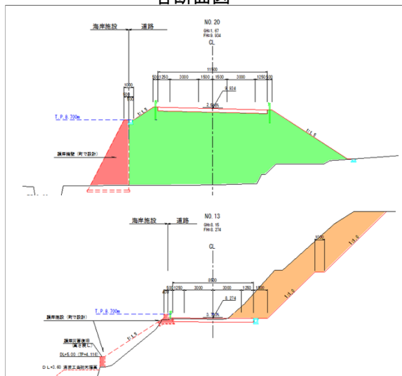
各断面図
