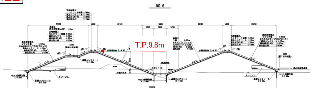
港川 標準断面図
