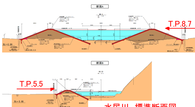
水尻川 標準断面図
