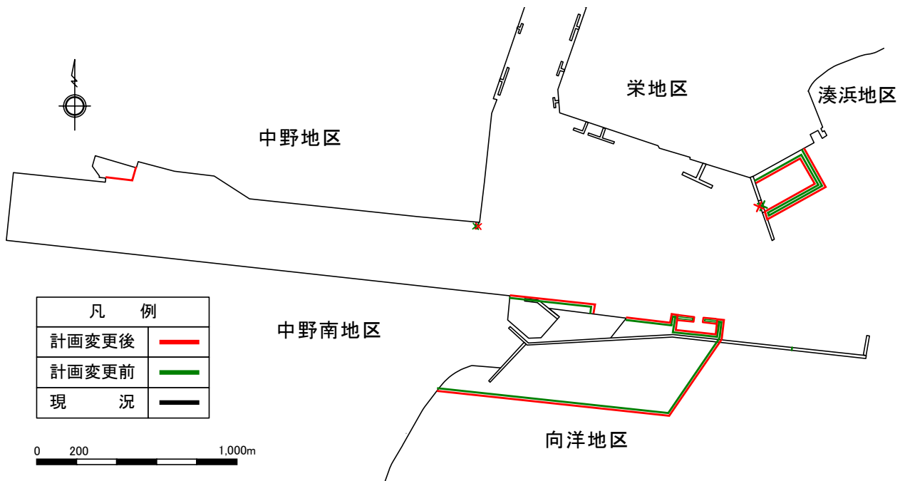
図Ⅷ-6-1(1) 新旧法線対照図(仙台港区)
