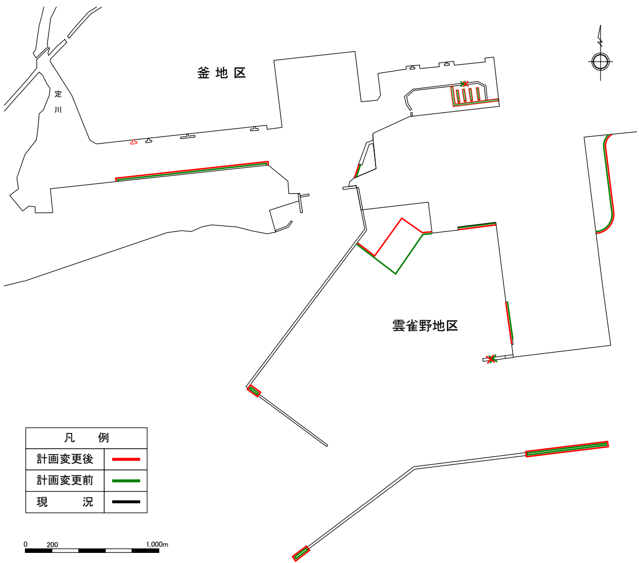
図Ⅷ-6-1(3) 新旧法線対照図(石巻港区)
