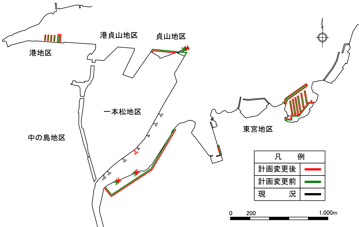
図Ⅷ-6-1(2) 新旧法線対照図(塩釜港区)
