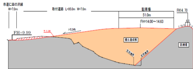
B - B' 断面
