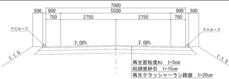
取付道路 標準断面図（案）
