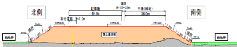
B - B' 断面
