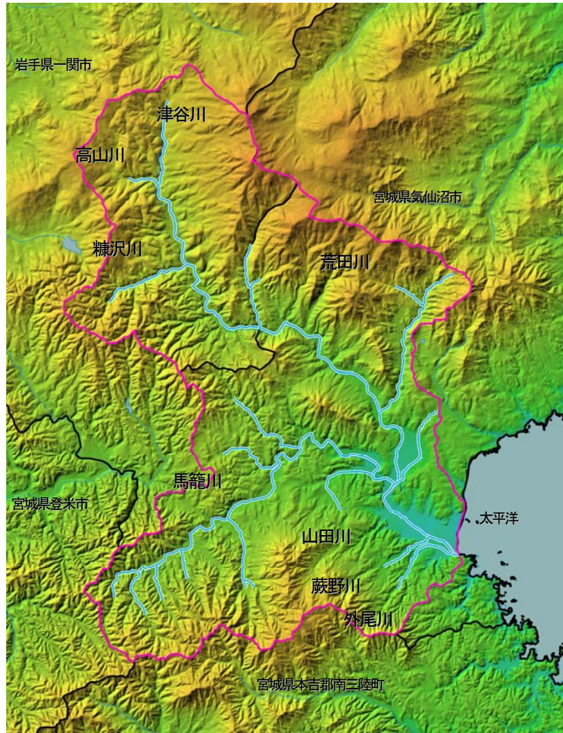
図 1-2 地形図
