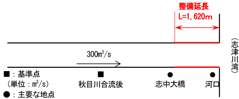
八幡川計画高水流量図
