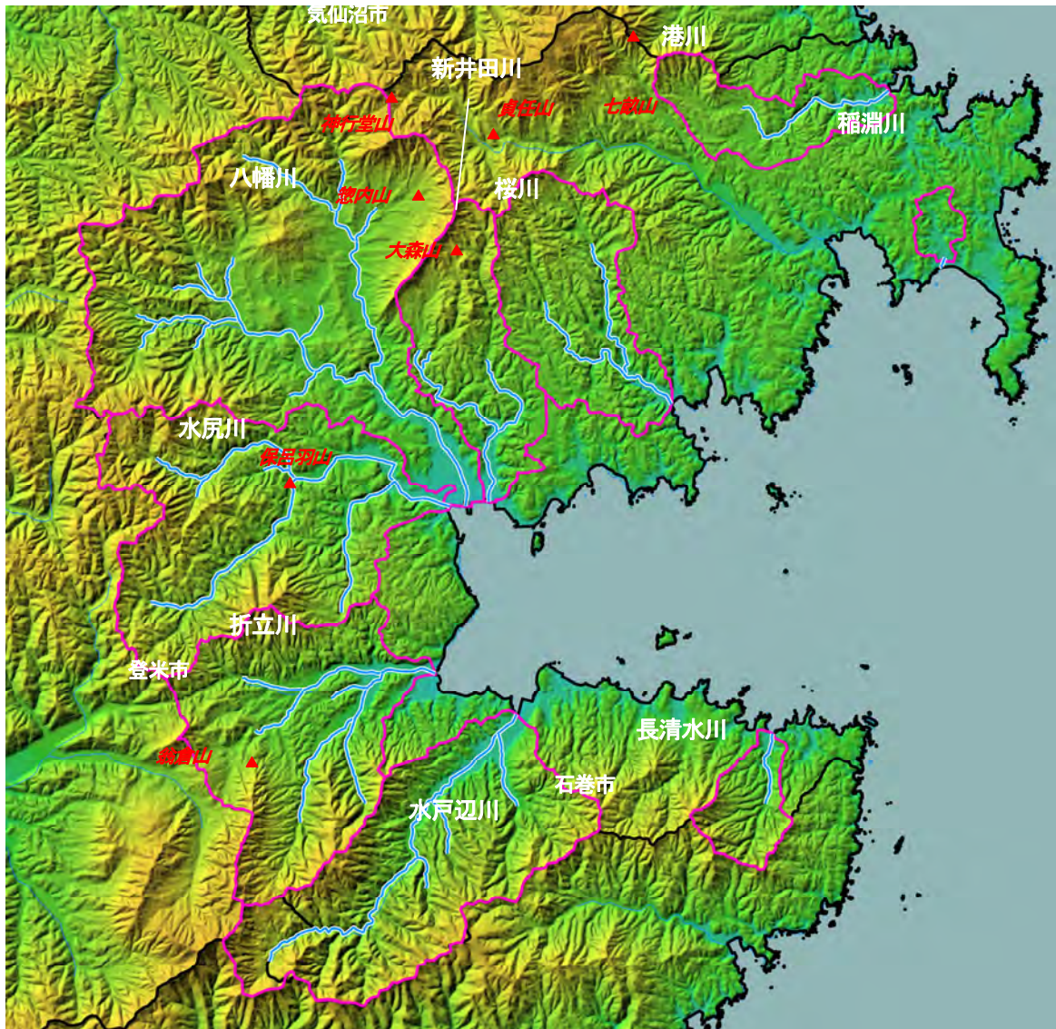
図 1-2 地形図
