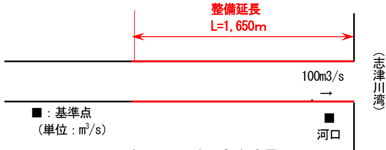
新井田川計画高水流量図
