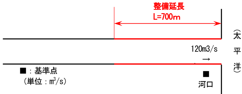
桜川計画高水流量図
