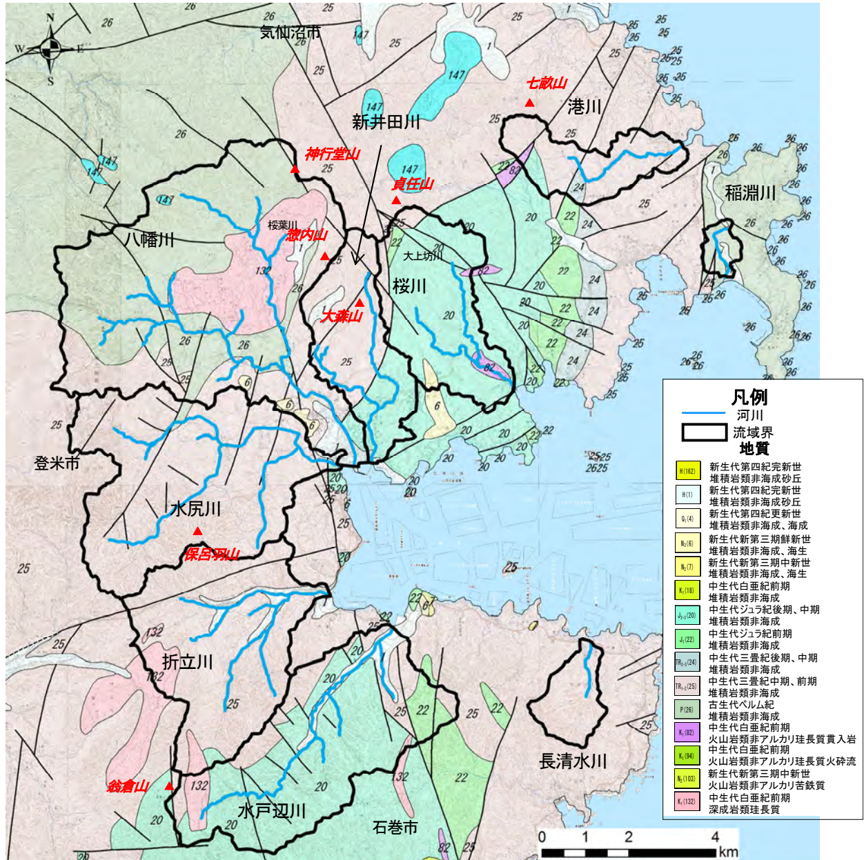
図 1-3 地質概略図
