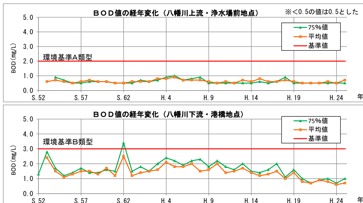
図 1-26 BOD 値の経年変化【八幡川：浄水場前、港橋】
