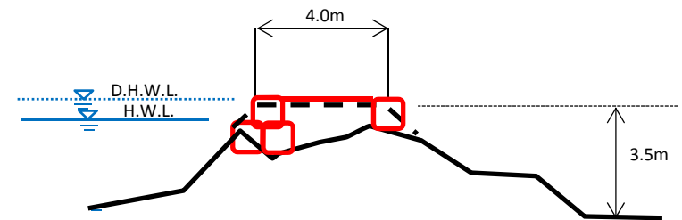
応急復旧標準断面図 (大型土のう・中詰土設置)
