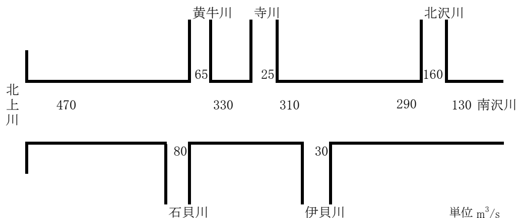
図 1-11 整備計画流量配分（南沢川）
