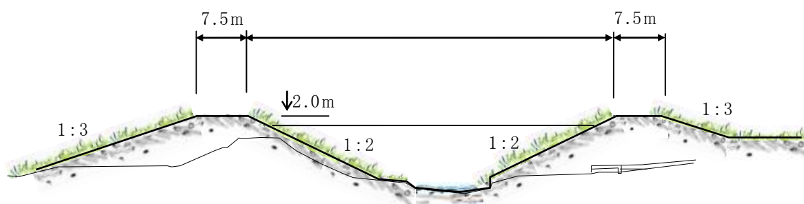
図 2-5 横断図（北上川合流点から 0.2km 上流付近）
