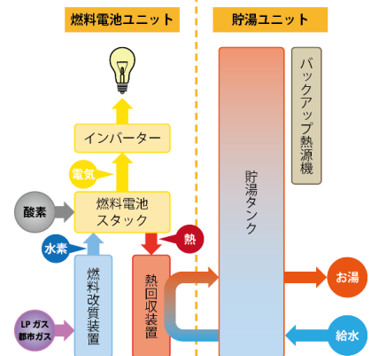
図 15：エネファームの仕組みのイメージ
