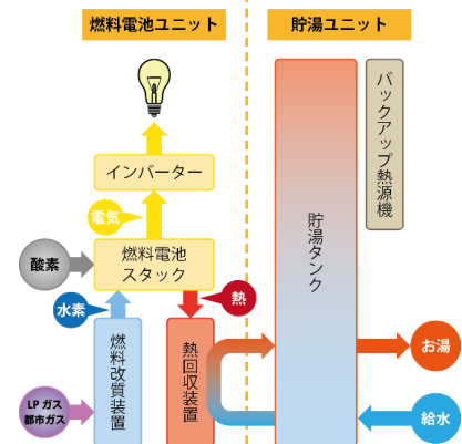
図 16：エネファームの仕組みのイメージ
