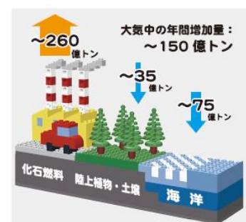
図 10：二酸化炭素の循環のイメージ
