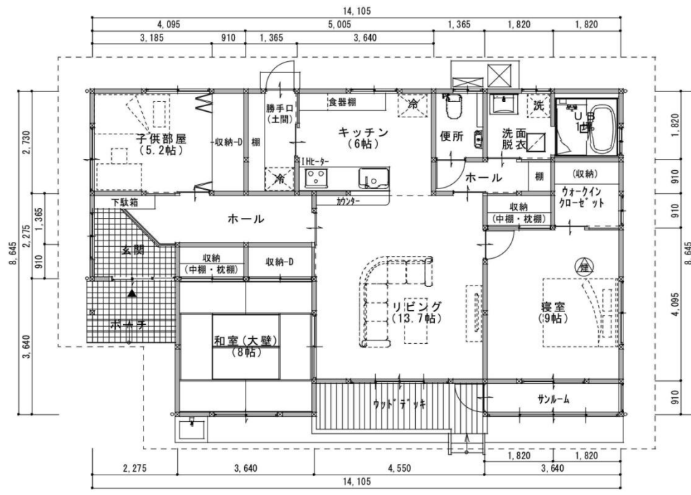
1階平面図
