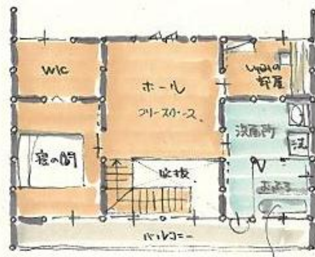
▲2階プラン
