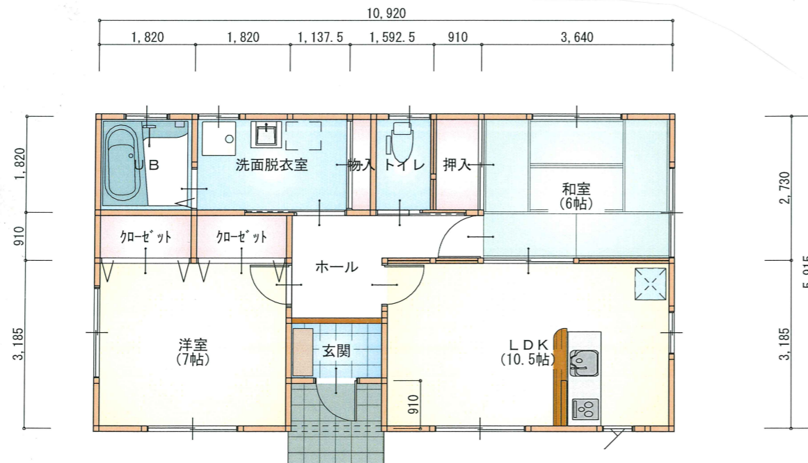
1階平面図
