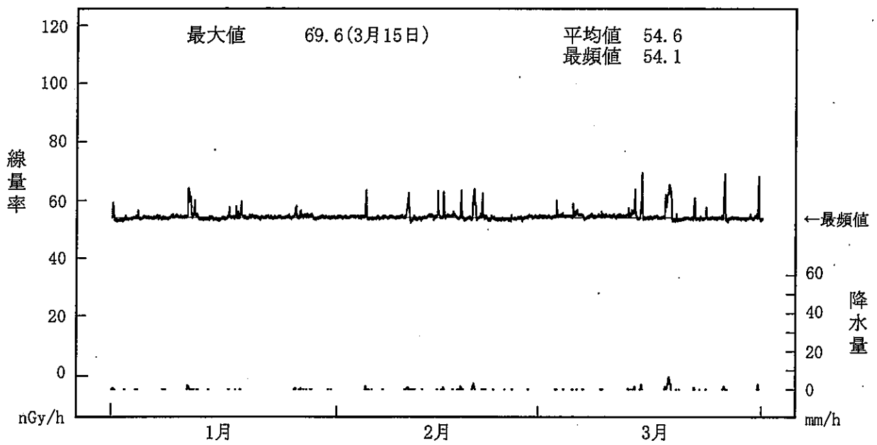
図-2-7 空間ガンマ線量率監視結果 (萩浜局)
