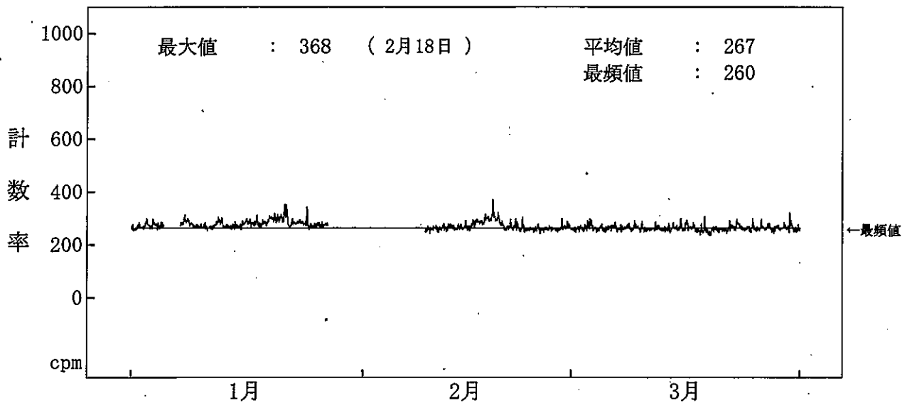
図一 2 - 1 3 海水(放水)中の全ガンマ線計数率監視結果(1号機放水口モニター(B))
