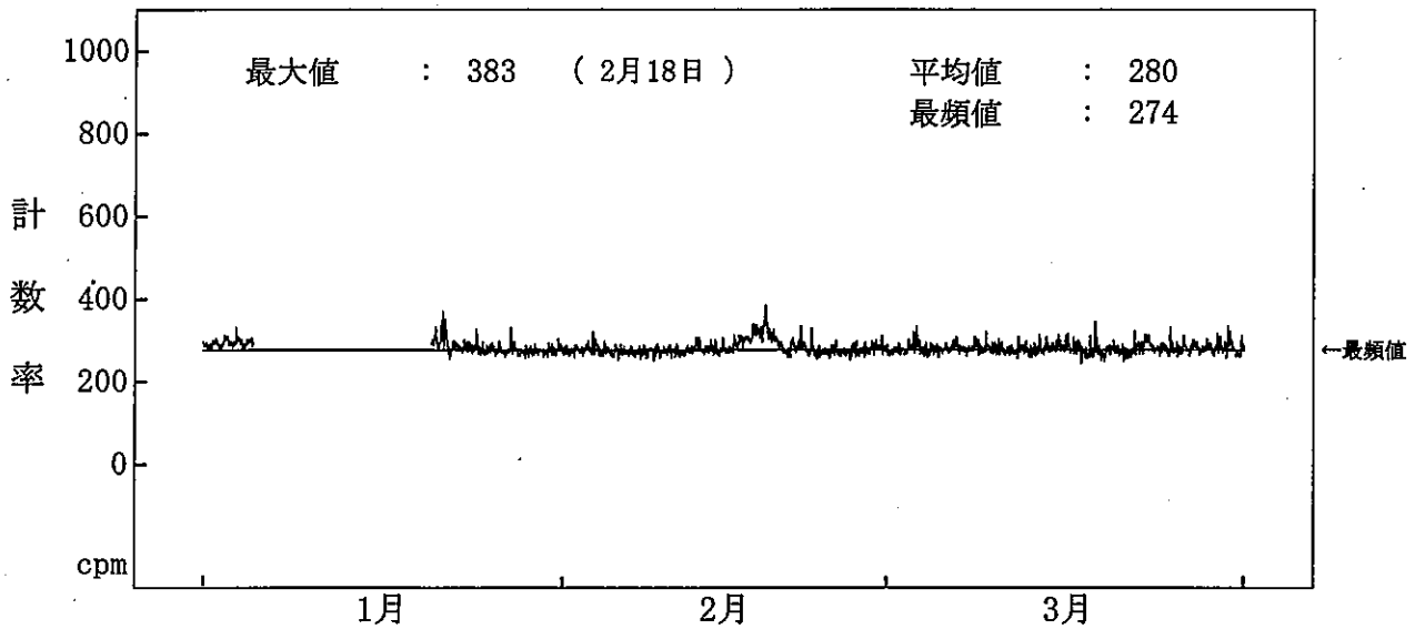
図一 2 - 1 2 海水(放水)中の全ガンマ線計数率監視結果(1号機放水口モニター(A))
