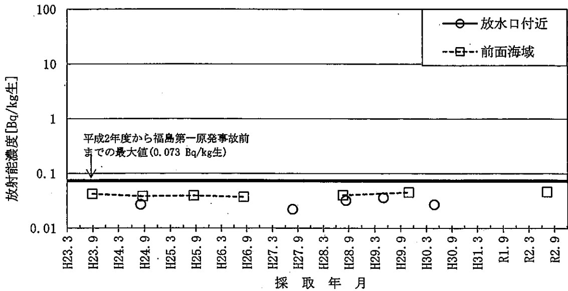
図-2-33 アラメのSr-90濃度の推移
