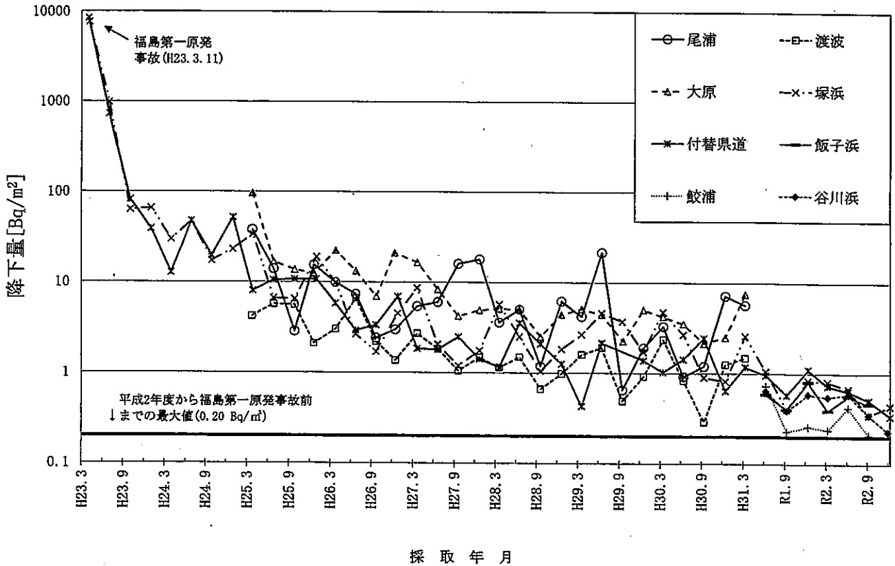
図-2-17 Cs-137の四半期間降下量の推移
