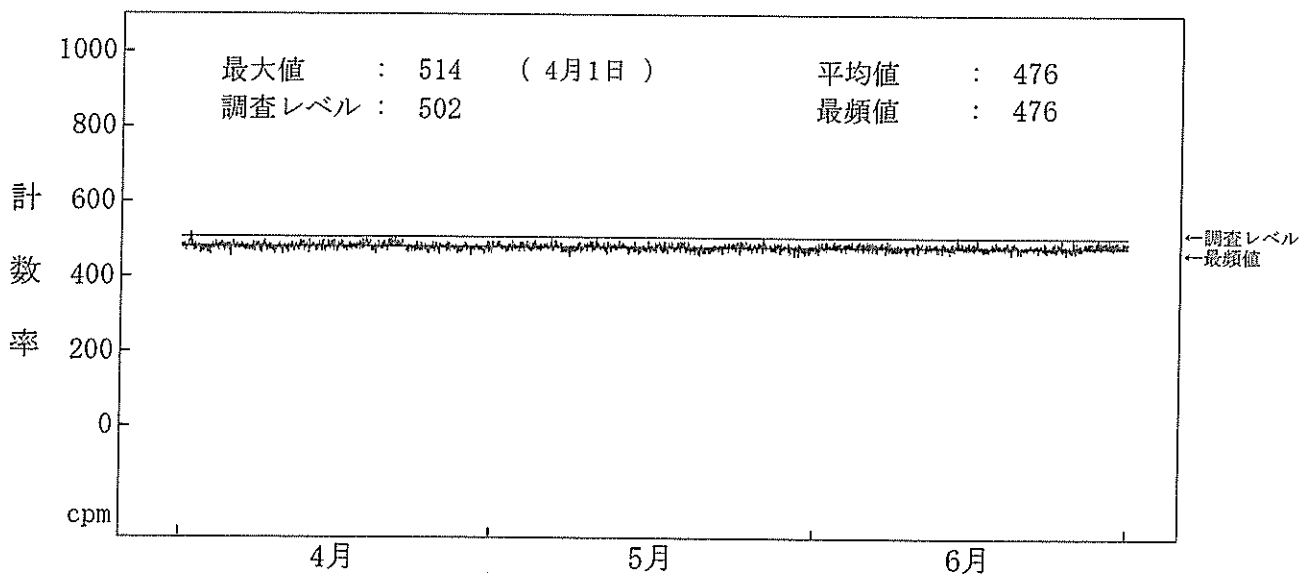
図一 2 - 1 5 海水(放水)中の全ガンマ線計数率監視結果(3号機放水口モニター) (注) 4月22日、5月27日及び6月11日の欠測は、定期点検によるものである。
