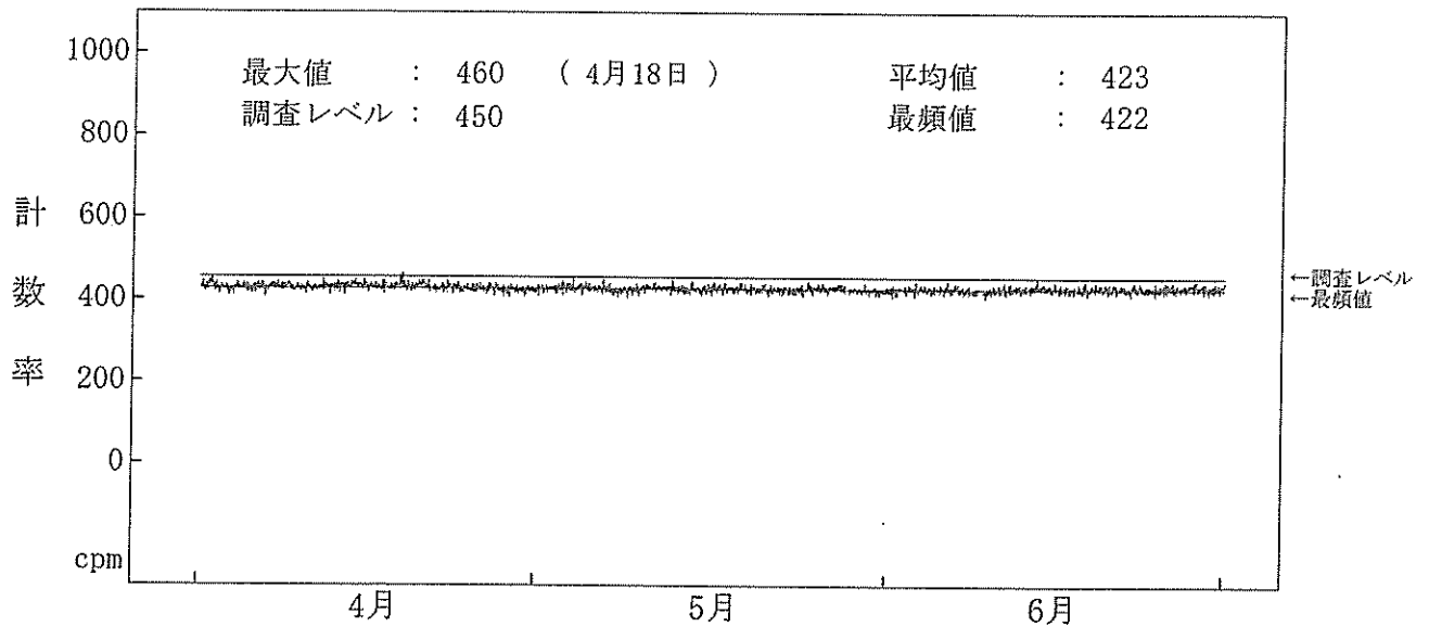
図一 2 - 1 4 海水(放水)中の全ガンマ線計数率監視結果(2号機放水口モニター) (注) 4月21日、5月28日及び6月9日の欠測は、定期点検によるものである。
