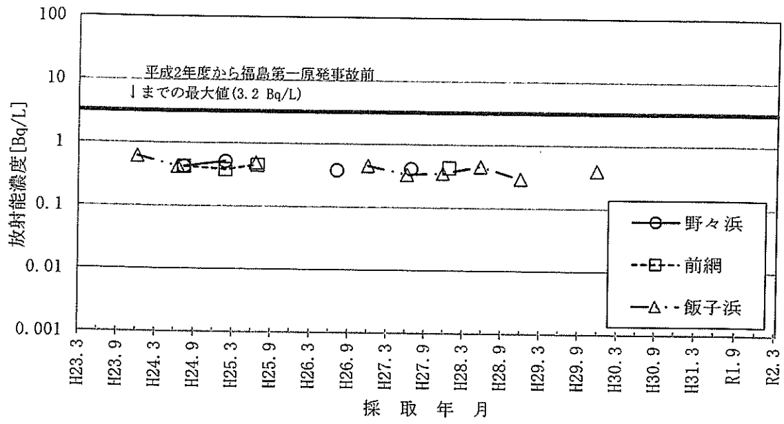
図-2-26 陸水のH-3濃度の推移
