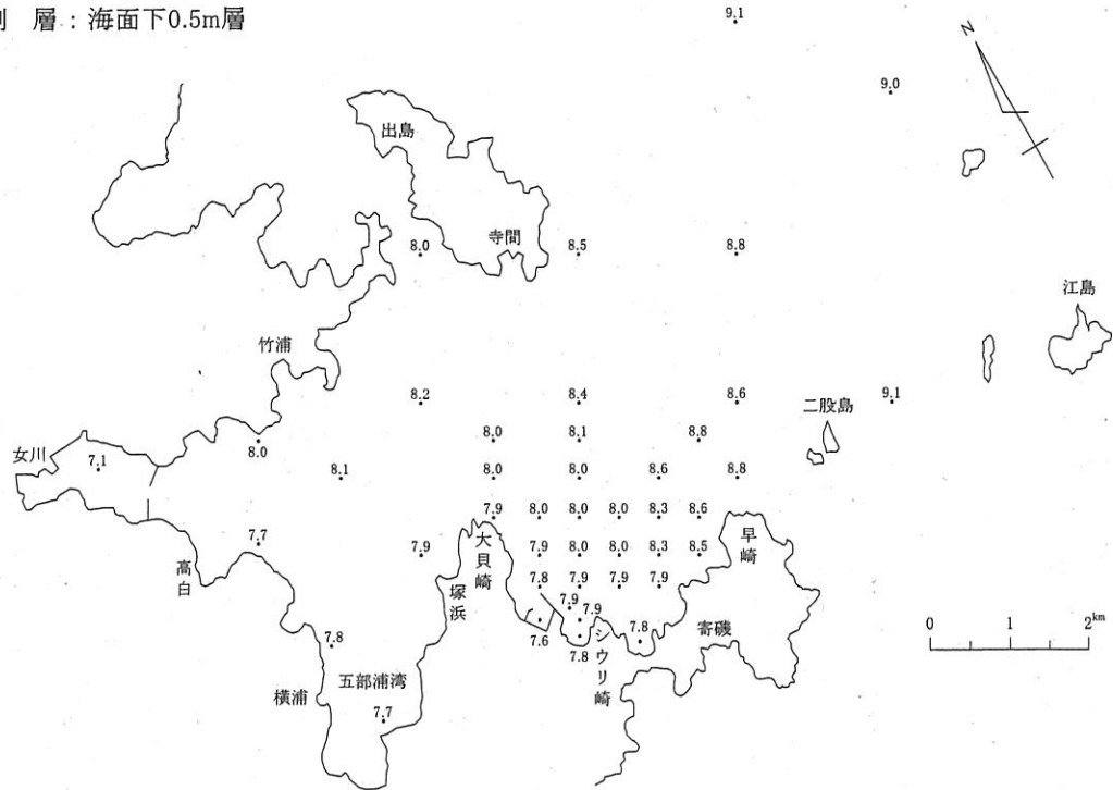
図-4-(1) 水温水平分布
