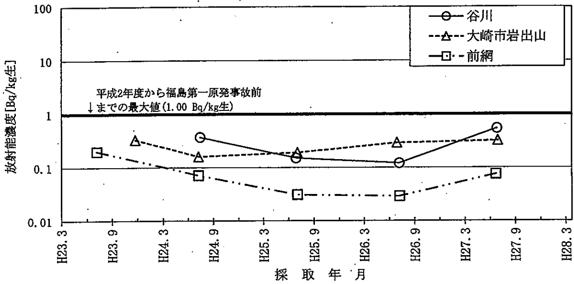
図-23 コモギのSr-90濃度の推移
