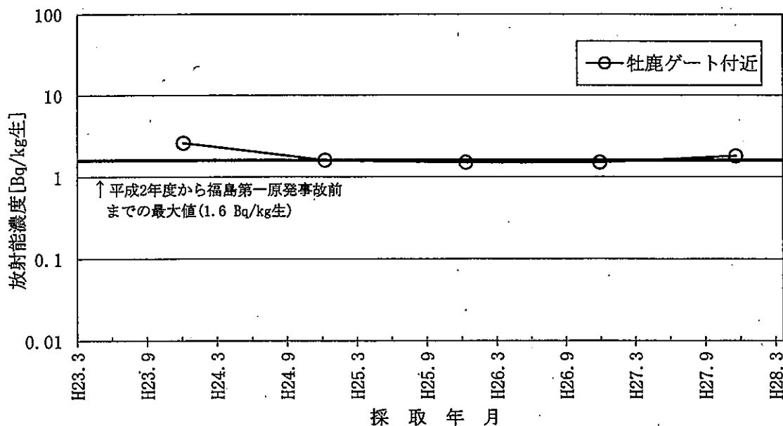
図-22 陸土のSr-90濃度の推移
