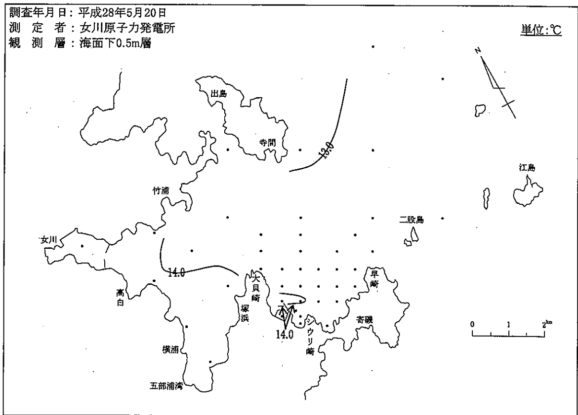
図-4-(2) 等温線
