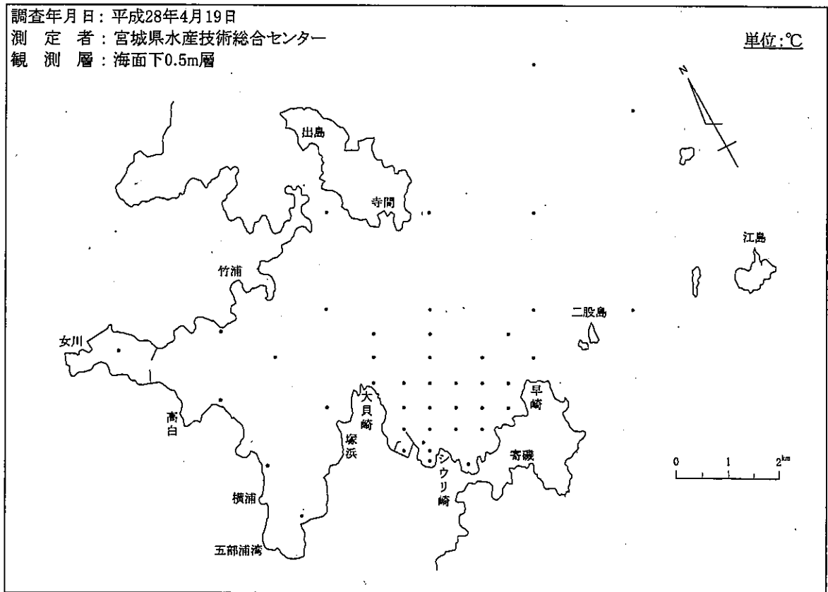
図-2-(2) 等温線
