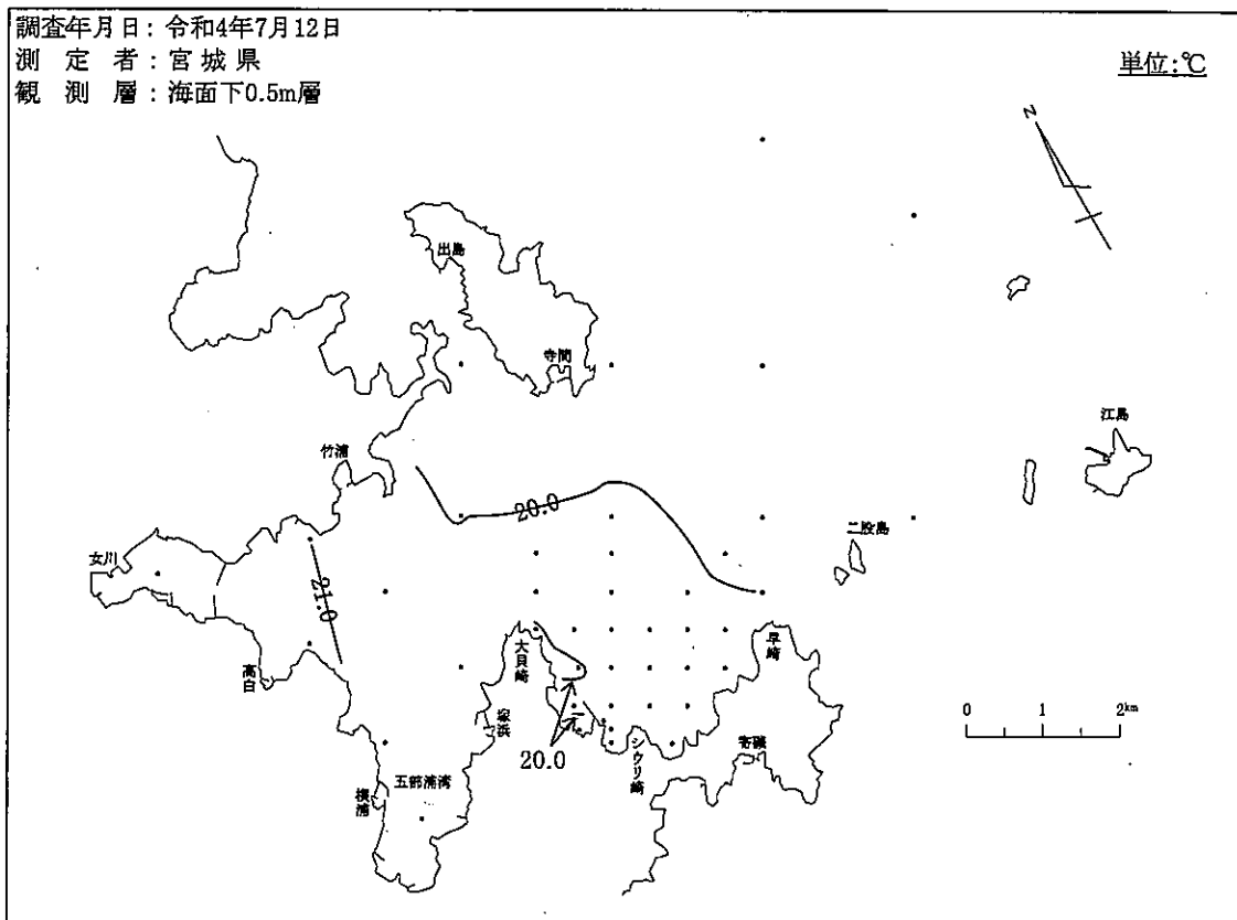
図-2-(2) 等温線
