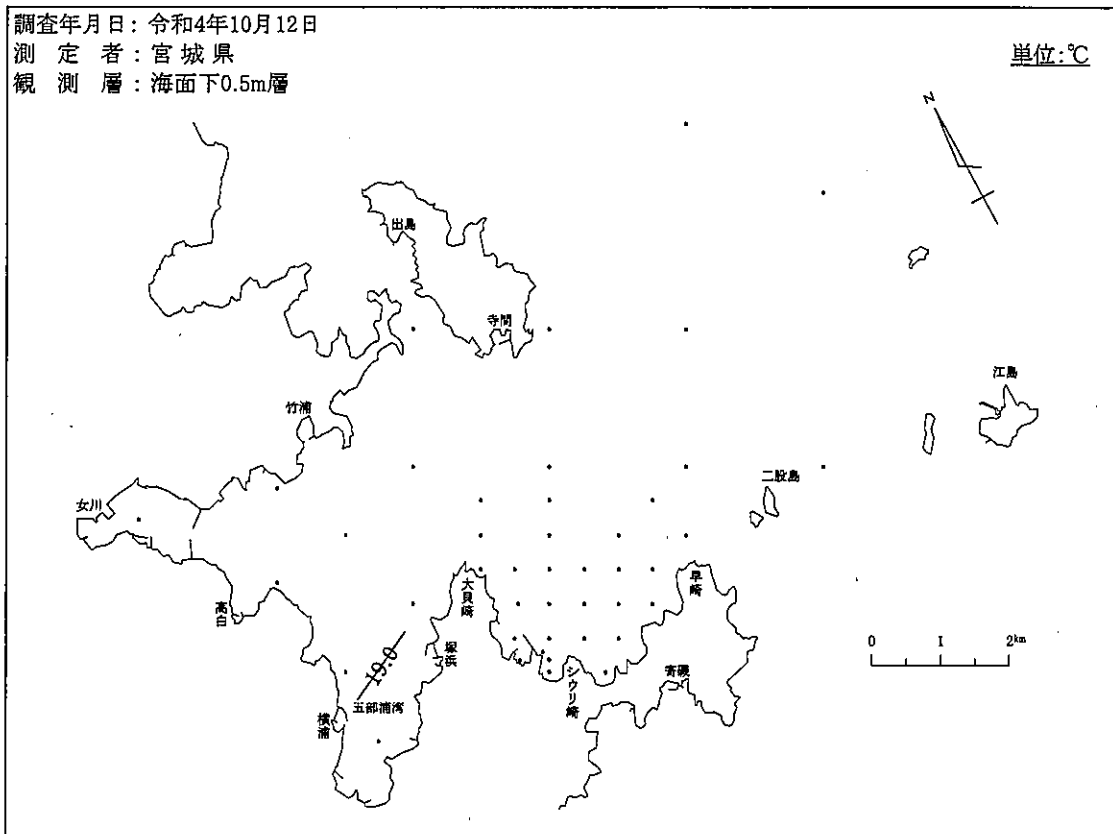
図-2-(2) 等温線
