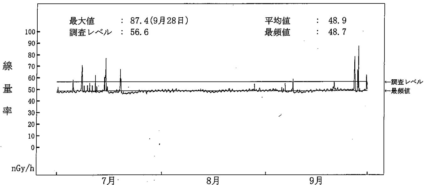
図-2-8 NaI(Tl)検出器による空間ガンマ線量率監視結果 (塚浜局)
