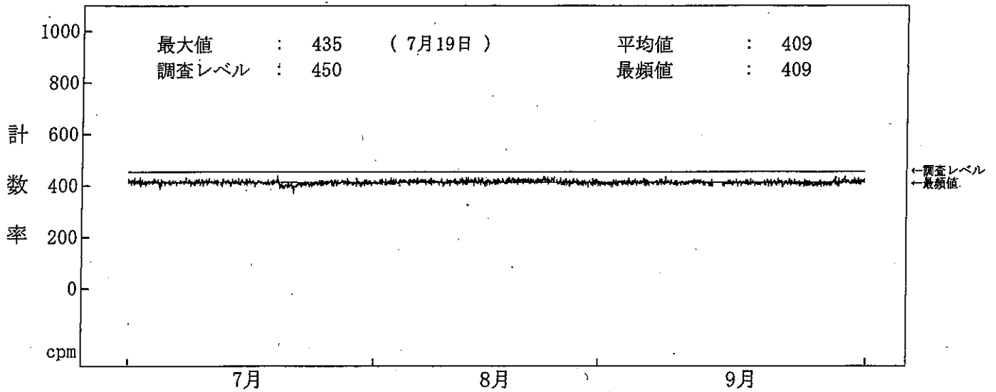
図-2-14 海水(放水)中の全ガンマ線計数率監視結果(2号機放水口モニター)
