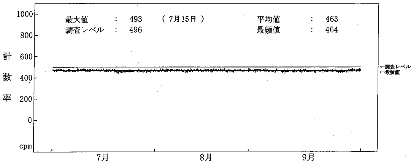
図-2-15 海水(放水)中の全ガンマ線計数率監視結果(3号機放水口モニター)
