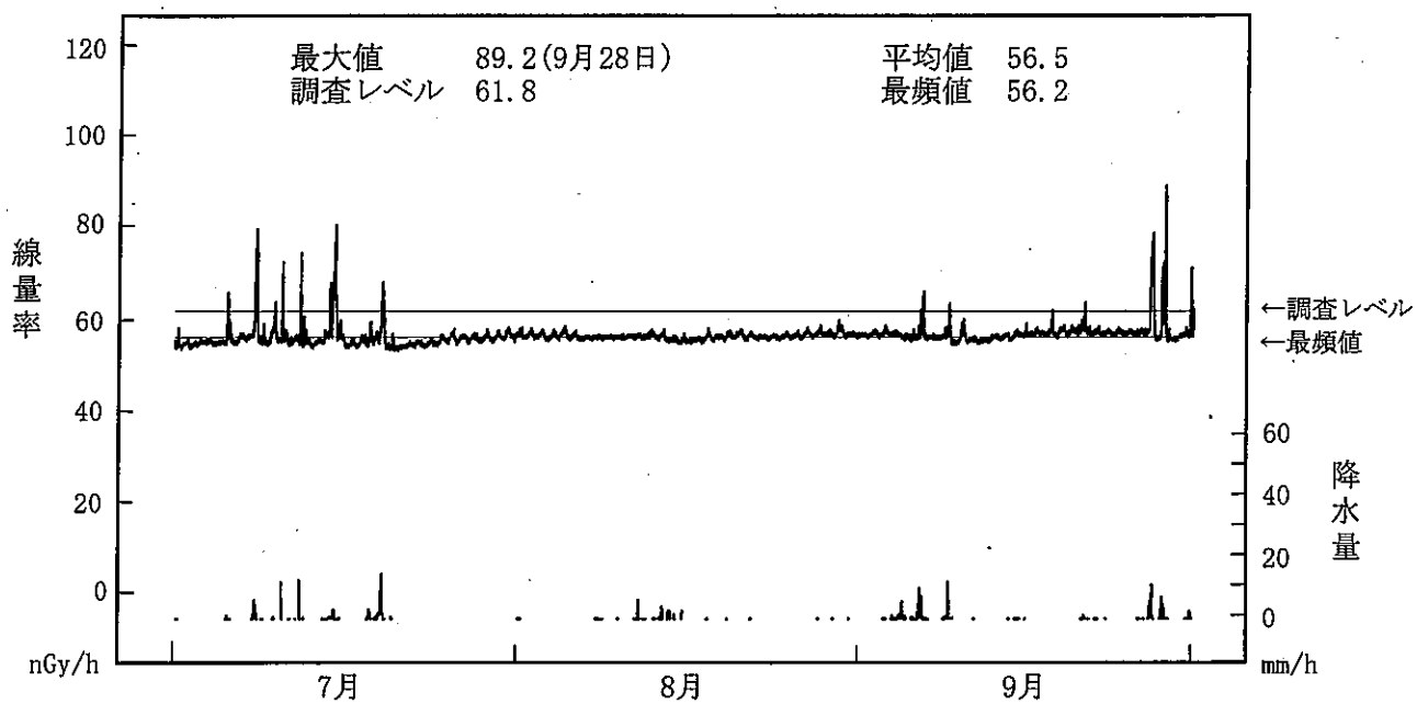
図一 2 - 7 NaI(Tl)検出器による空間ガンマ線量率監視結果 (荻浜局)
