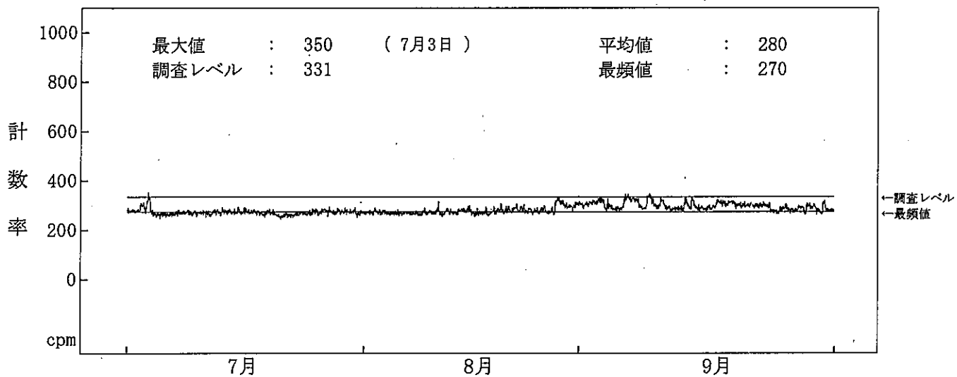
図-2-13 海水(放水)中の全ガンマ線計数率監視結果(1号機放水口モニター(B))
