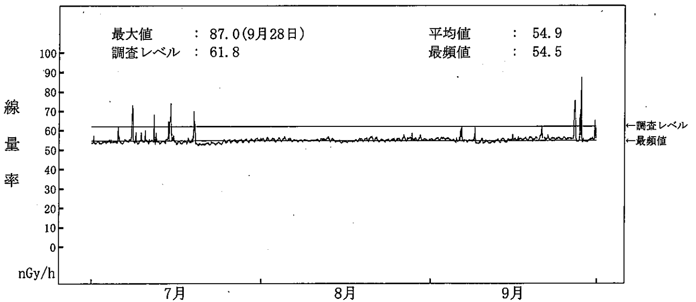
図-2-11 NaI(Tl)検出器による空間ガンマ線量率監視結果 (前網局)
